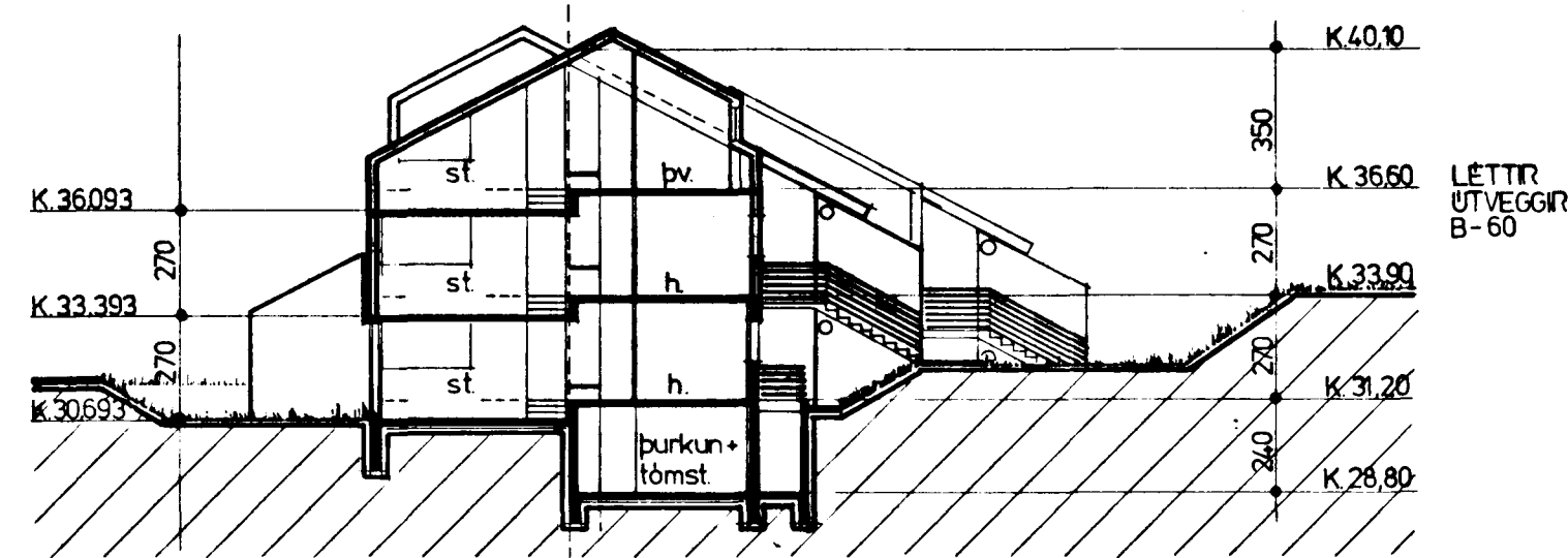
sneiding b-b
