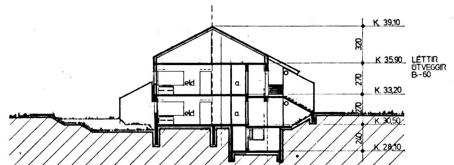
sneiding a-a
