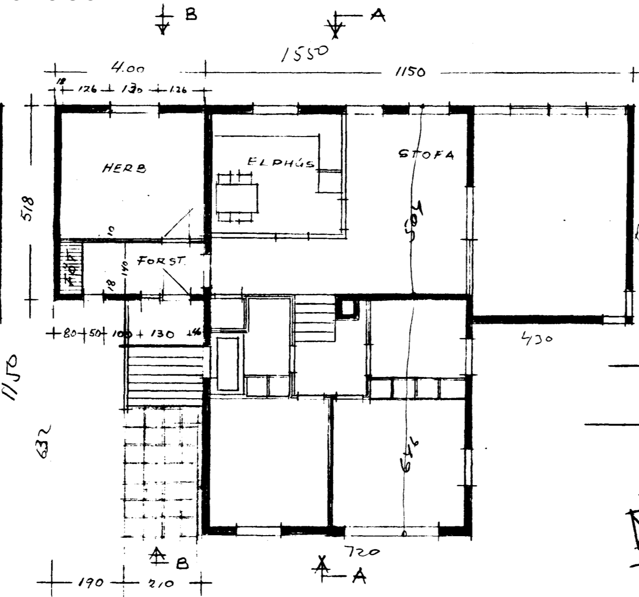
2. HÆÐ
