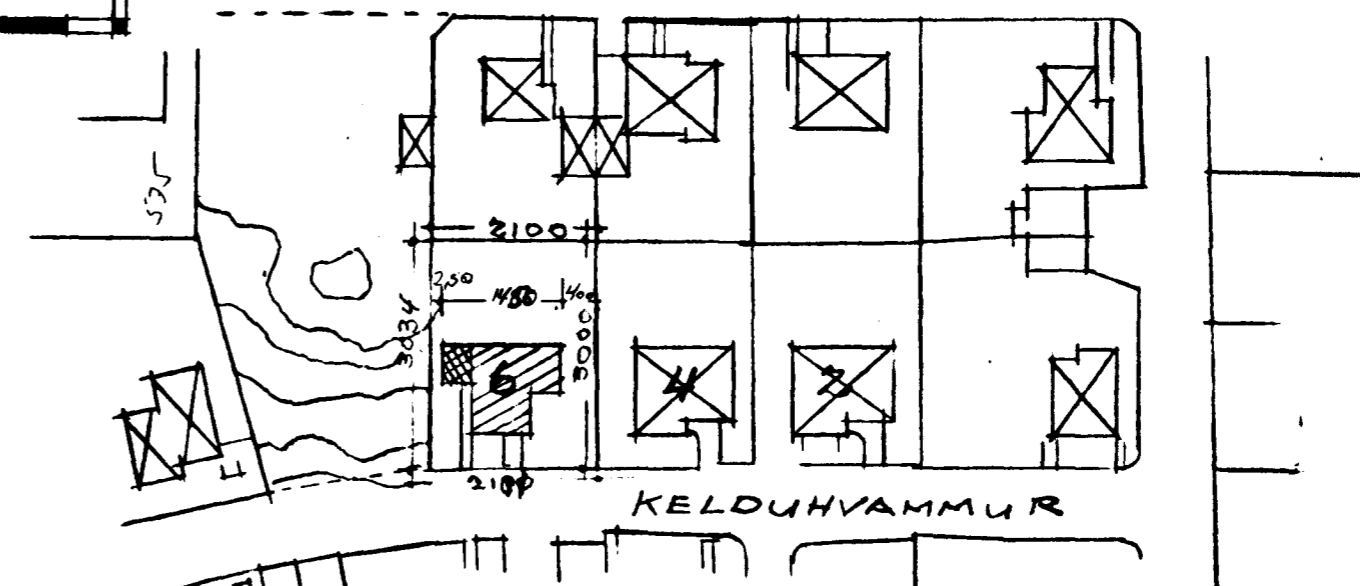
AFSTÖÐUMYND MKV: 1:1000
