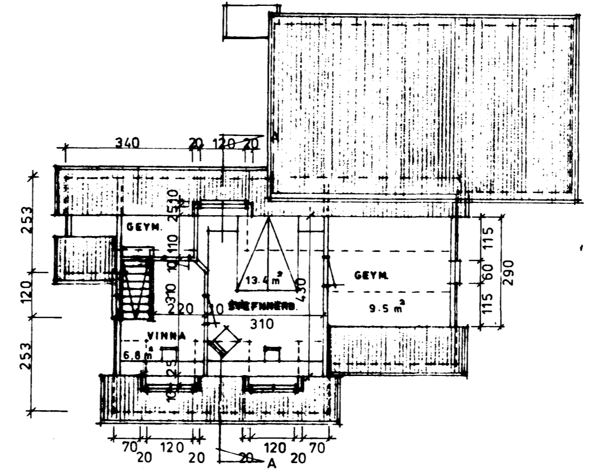
RIS M. 1:100
