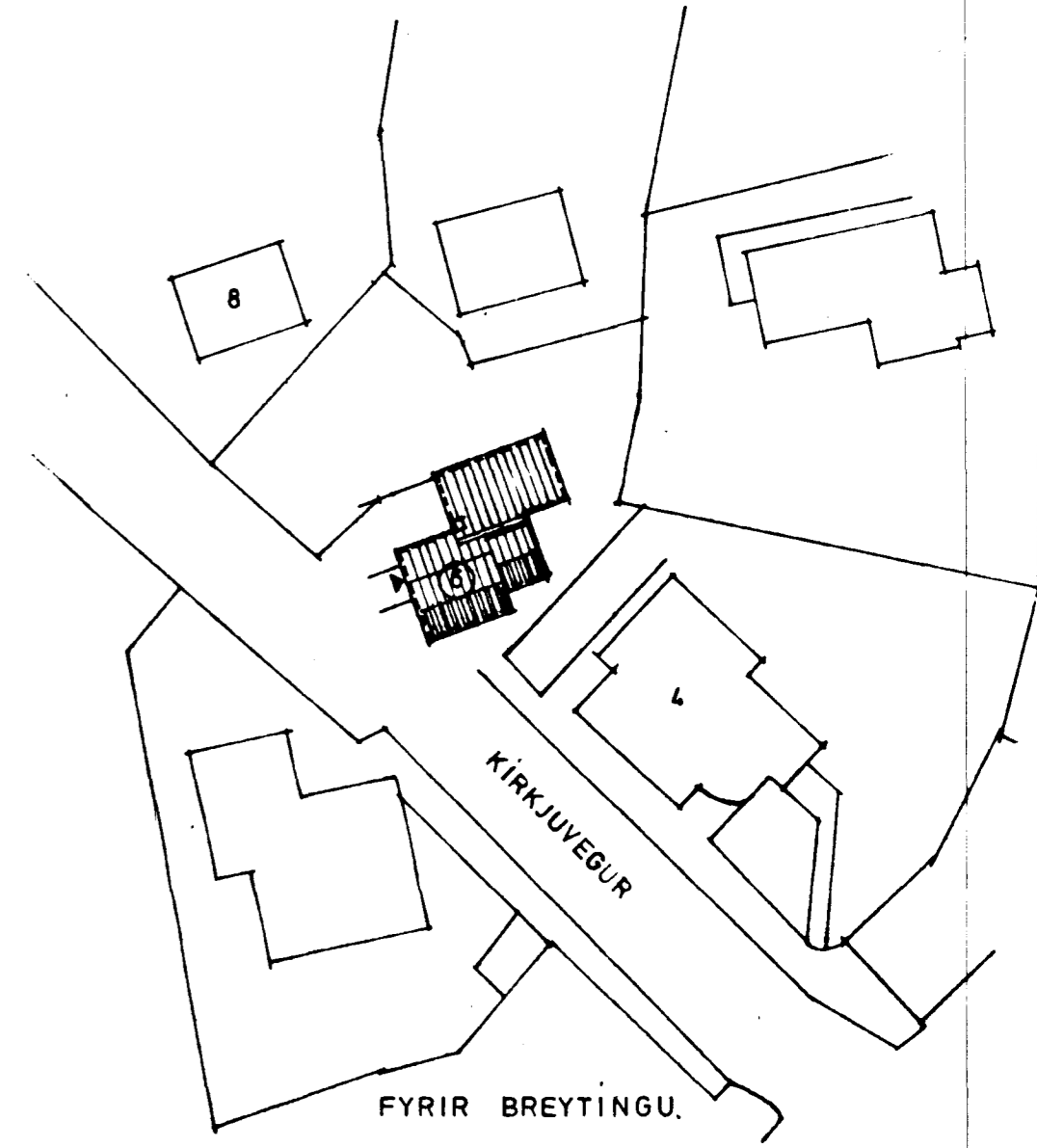
AFSTÖÐUMYND M. 1:500.
