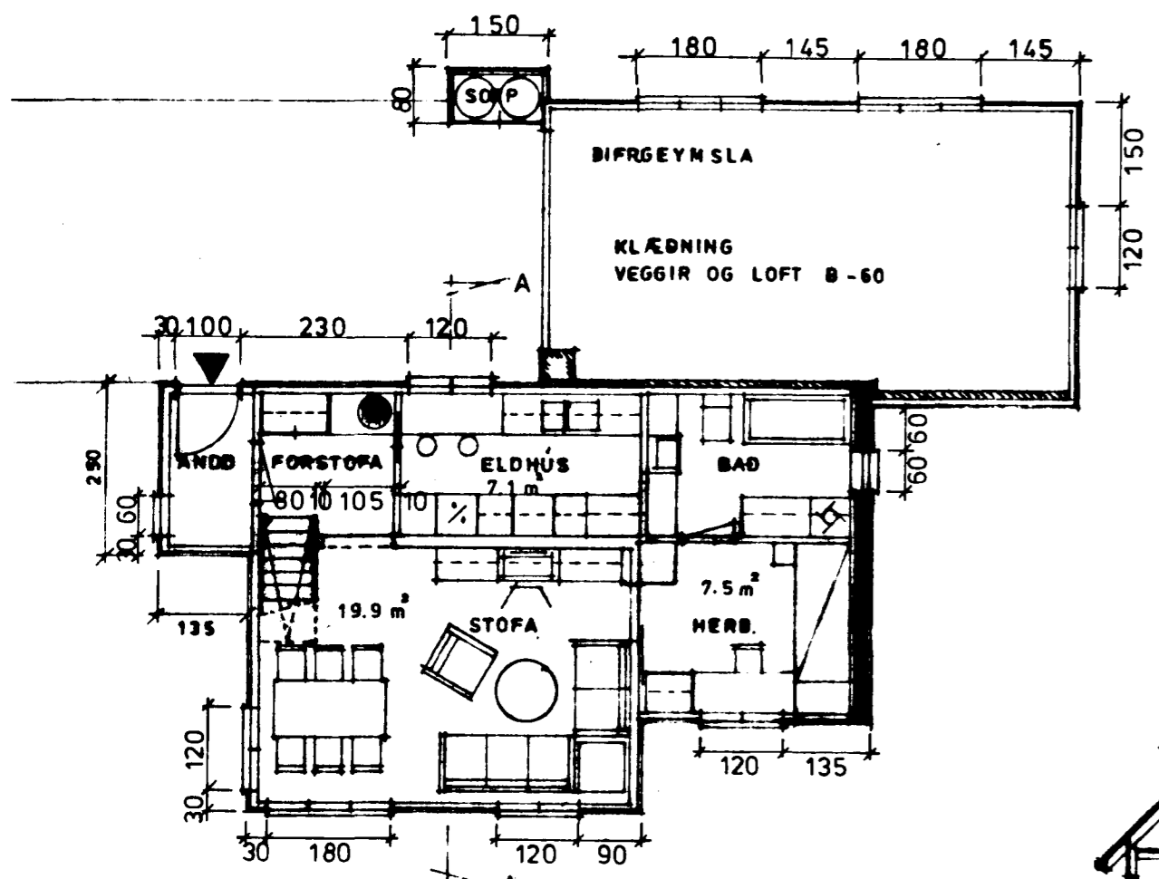
HÆÐ M. 1:100.
