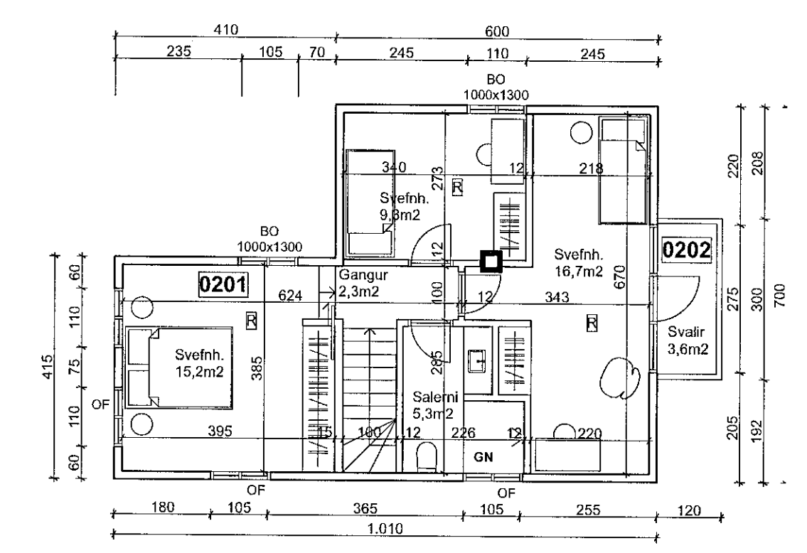
Grunnmynd 2.Hæð 1:100
