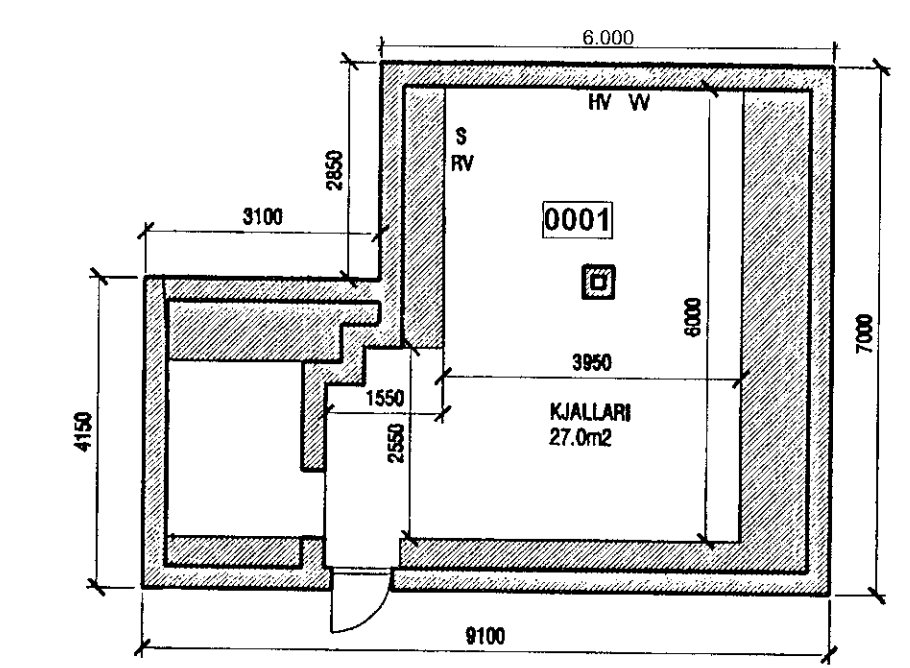
Grunnmynd Kjallari 1:100
