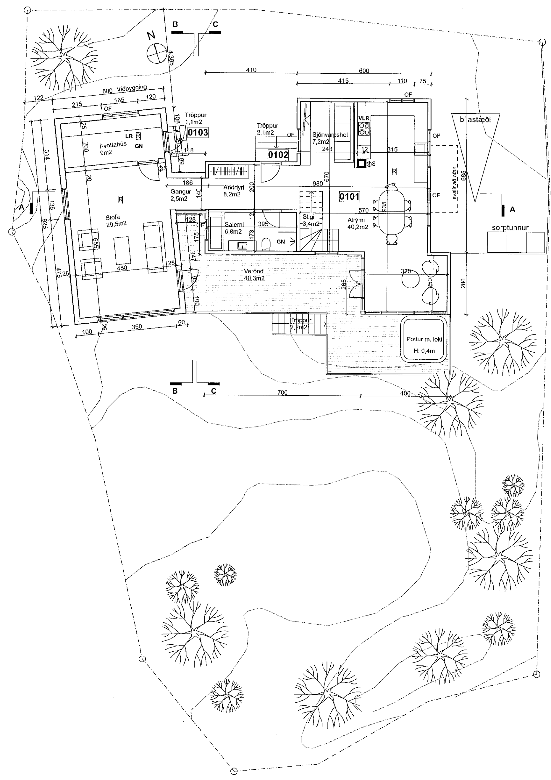
Grunnmynd 1.hæð 1:100
