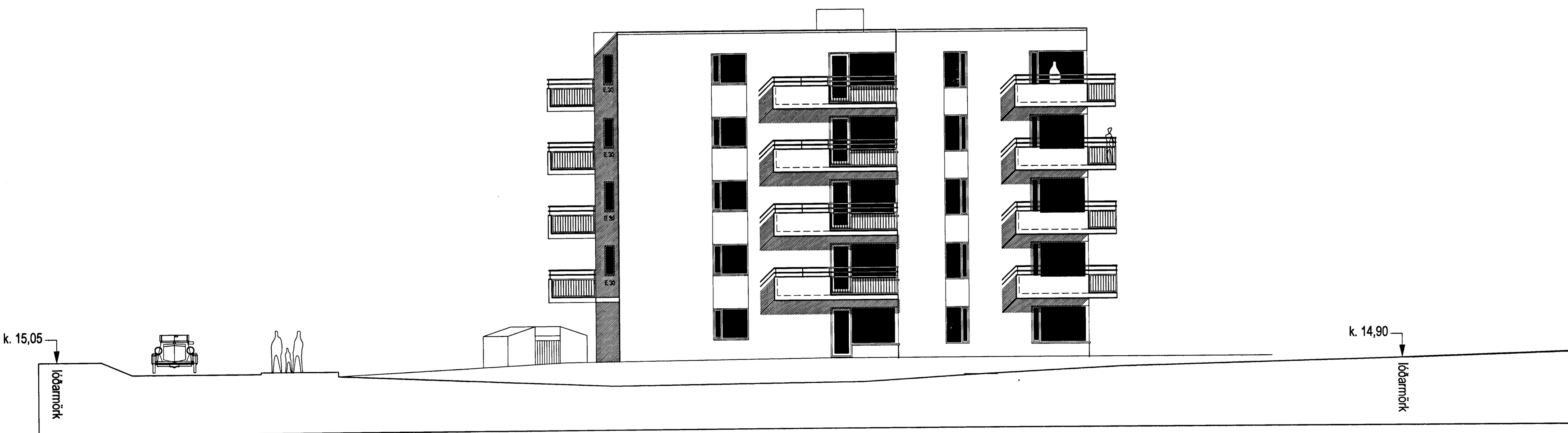
ÚTLIT 1:100 VESTUR HLIÐ
