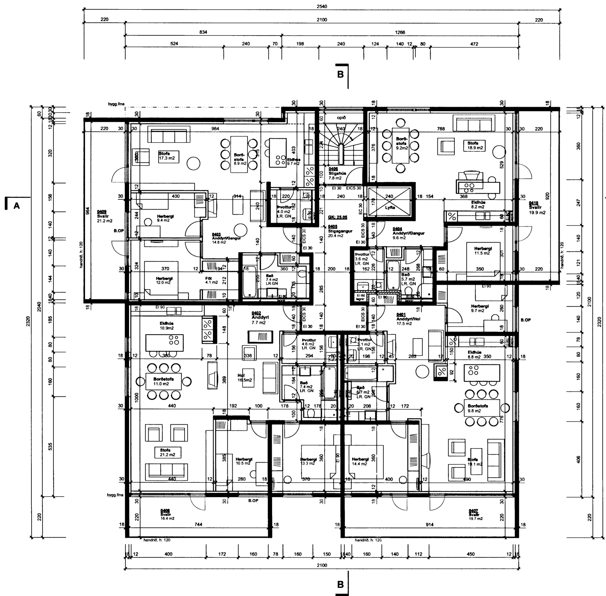
GRUNNMYND 4. HÆÐAR
