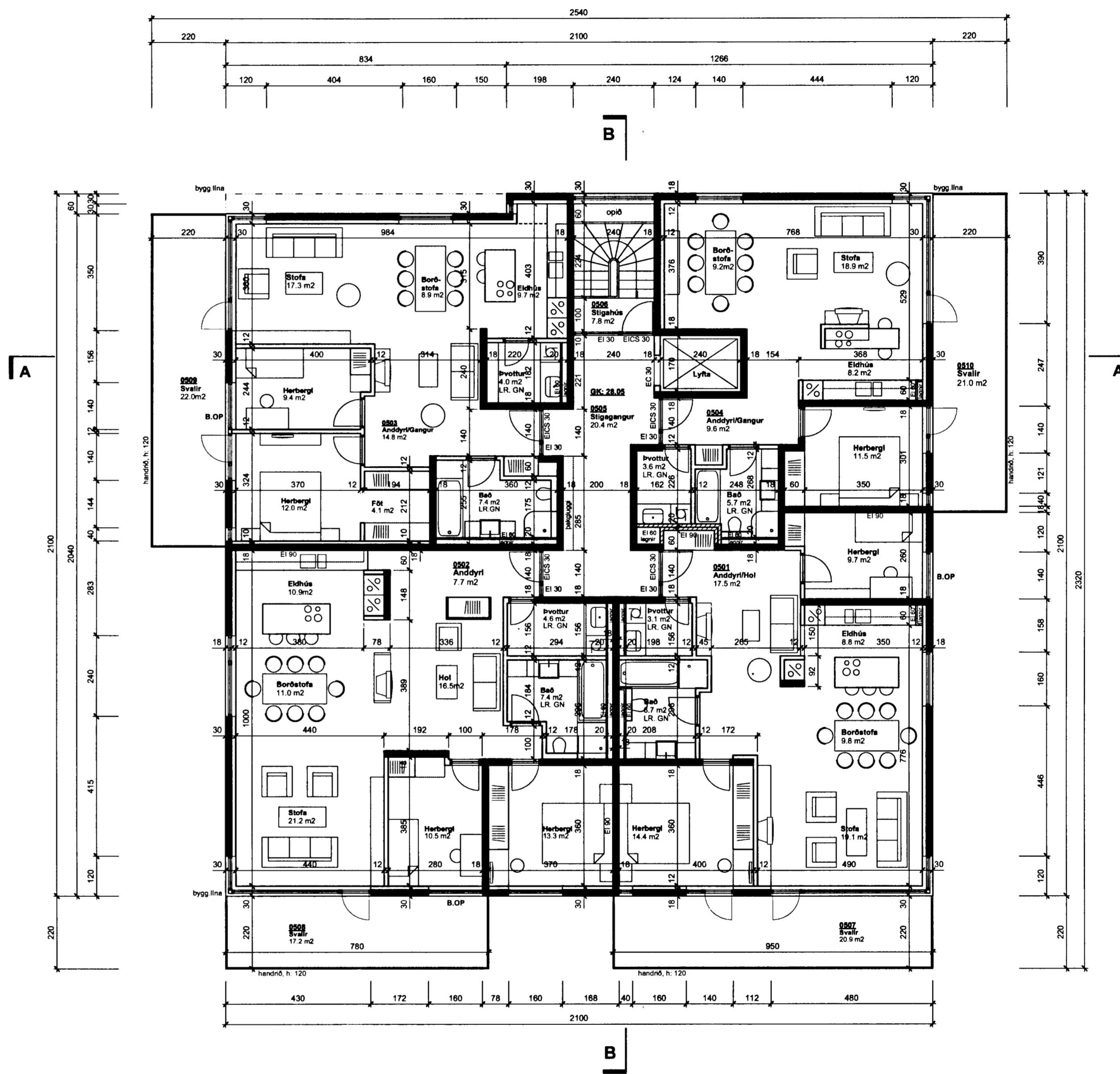
GRUNNMYND 5. HÆÐAR
