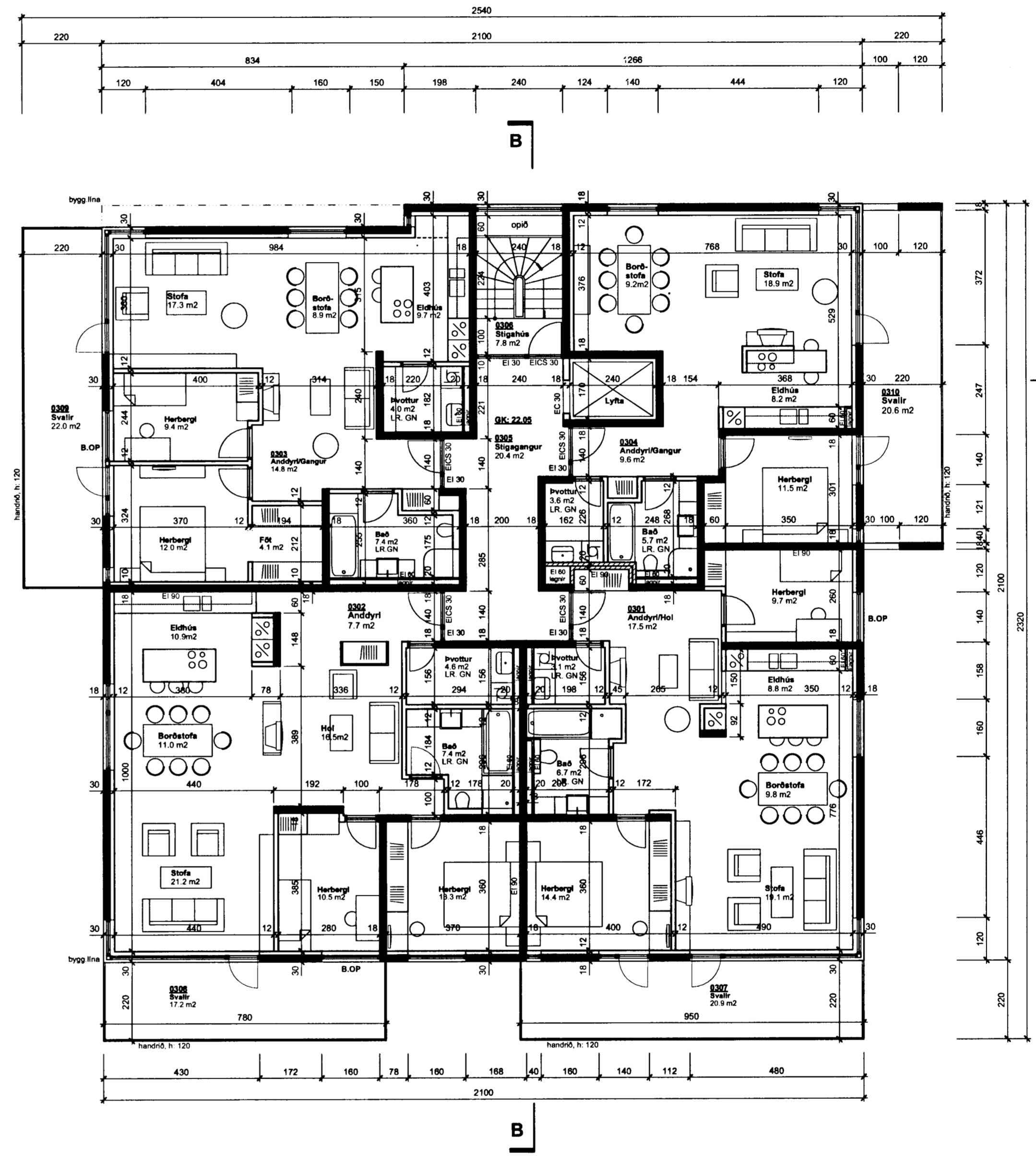
GRUNNMYND 3. HÆÐAR
