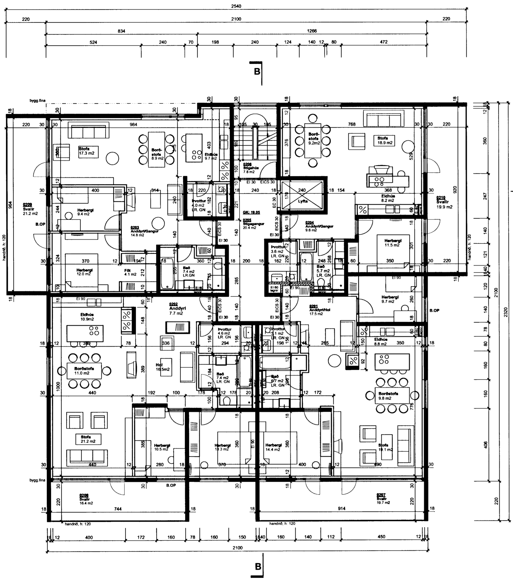
GRUNNMYND 2. HÆÐAR
