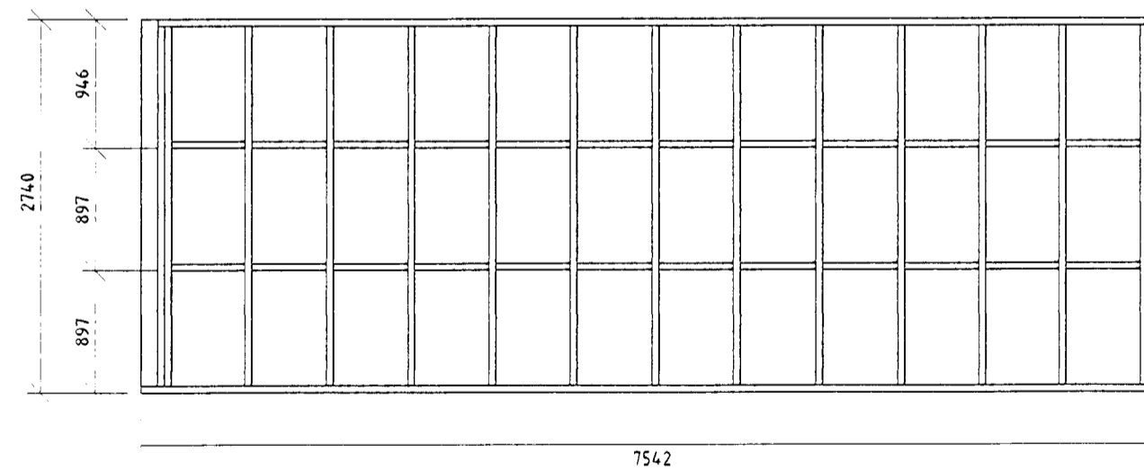
VEGGJAGRIND VESTURHLIÐAR
