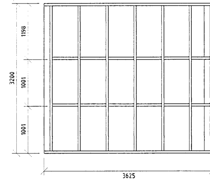
VEGGJAGRIND AUSTURHLIÐAR
