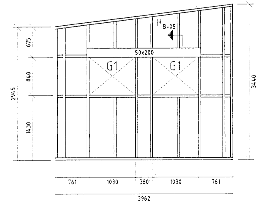
VEGGJAGRIND SUÐURHLIÐAR
