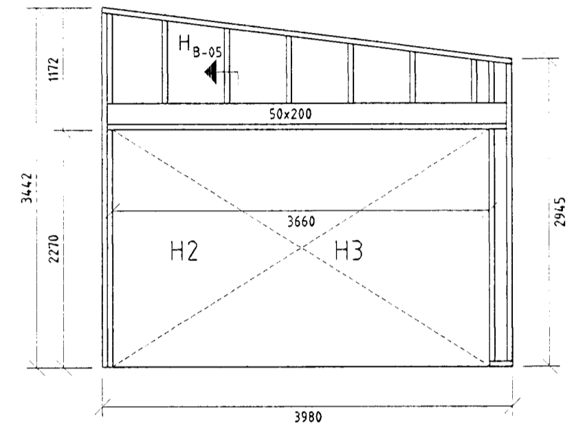
VEGGJAGRIND NORÐURHLIÐAR
