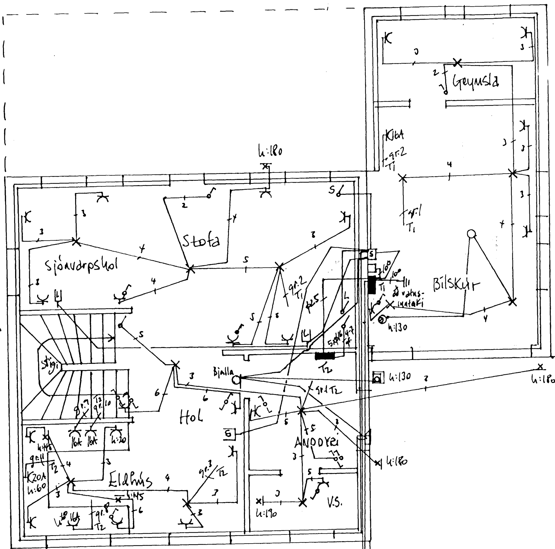
GRUNNMÝND 1. Höfðar 1:50
