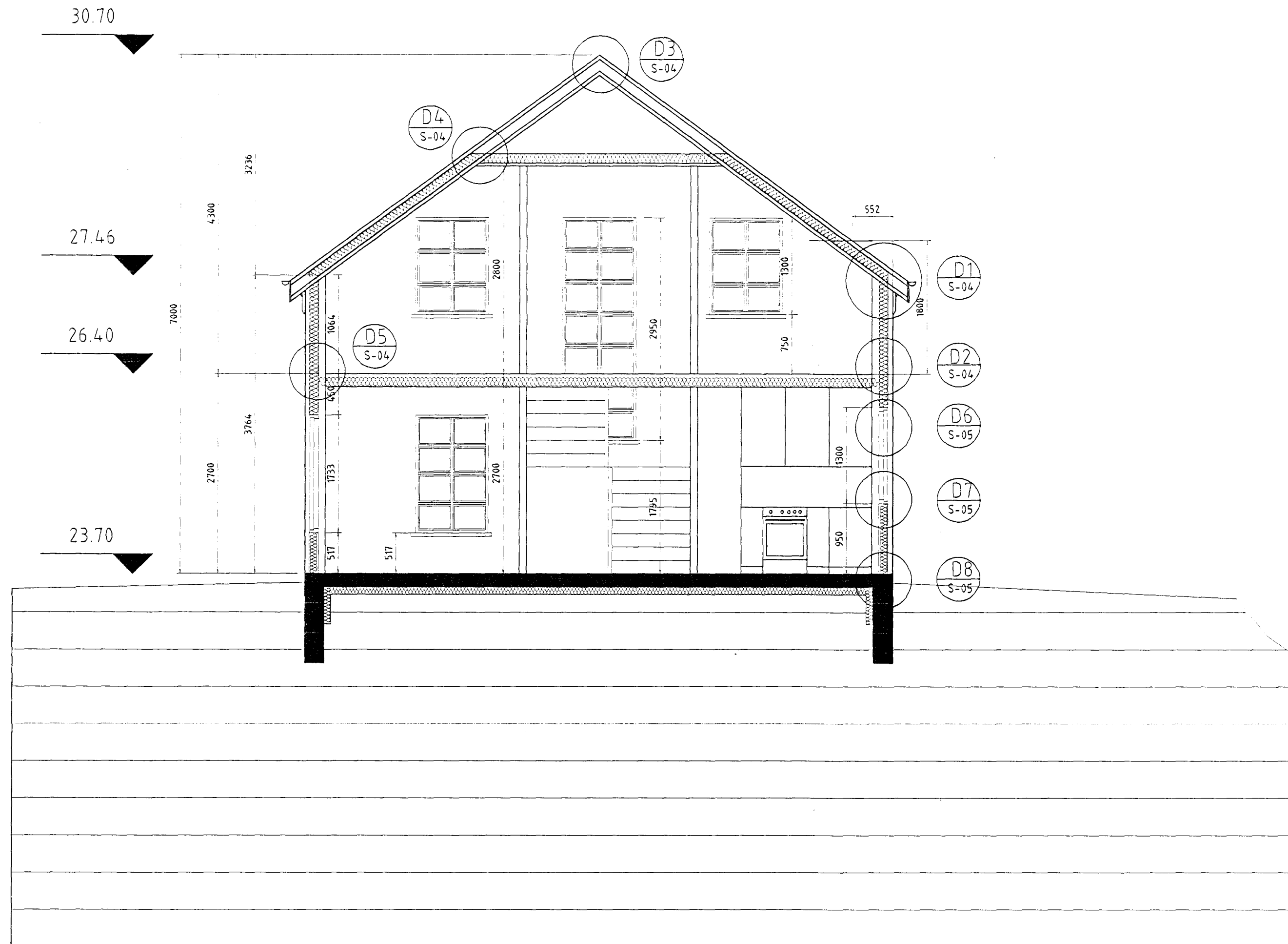
SNEIÐING A-A
