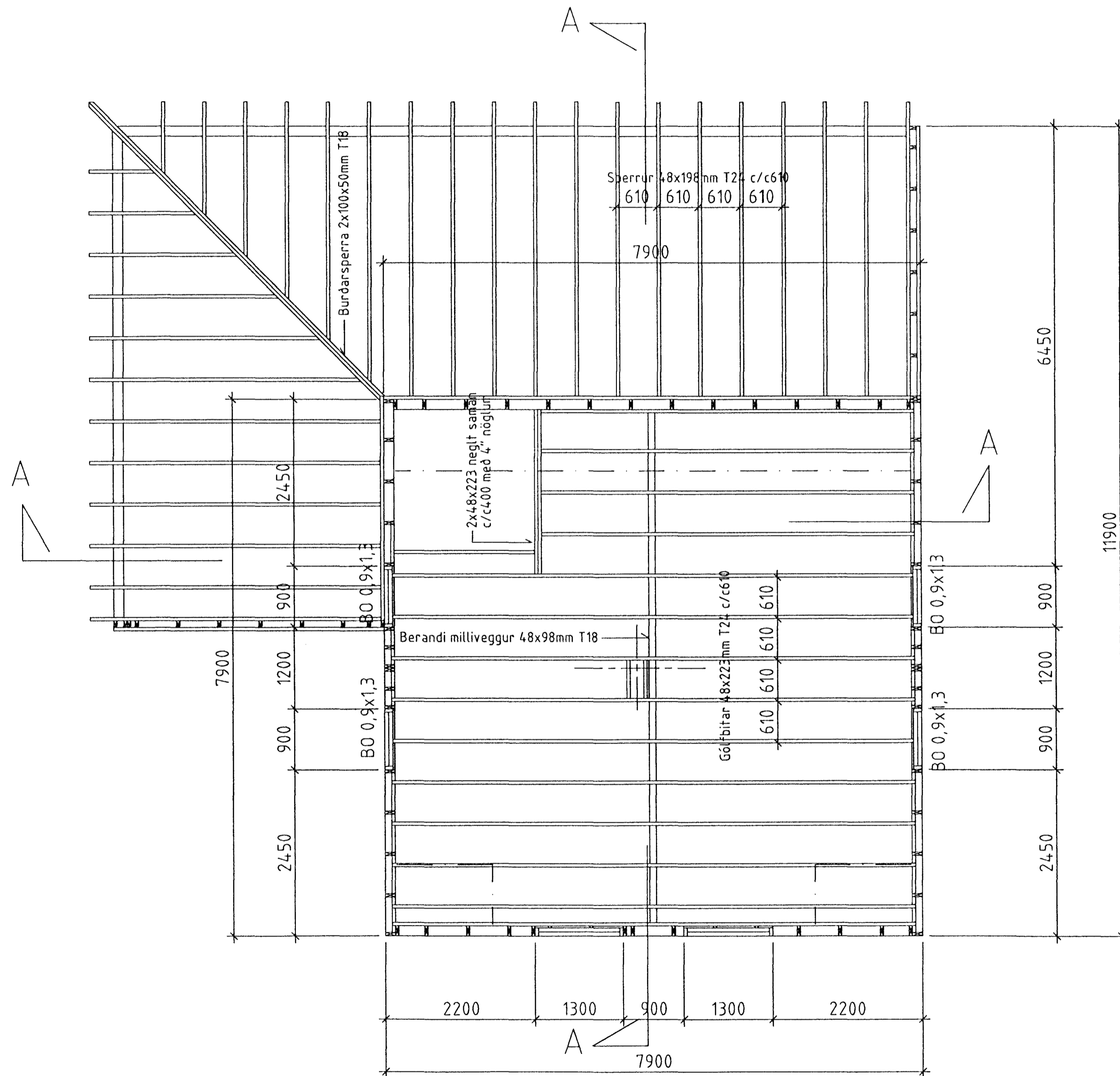
2. HÆÐ Gólfbitar og sperrur á lágbyggingu
