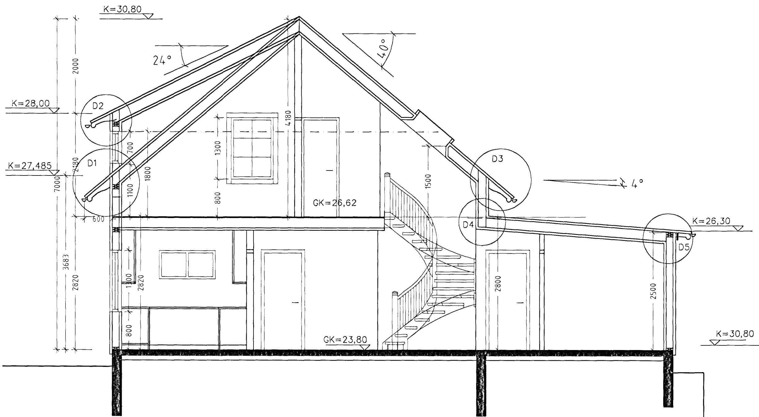
Sneiðing A-A
