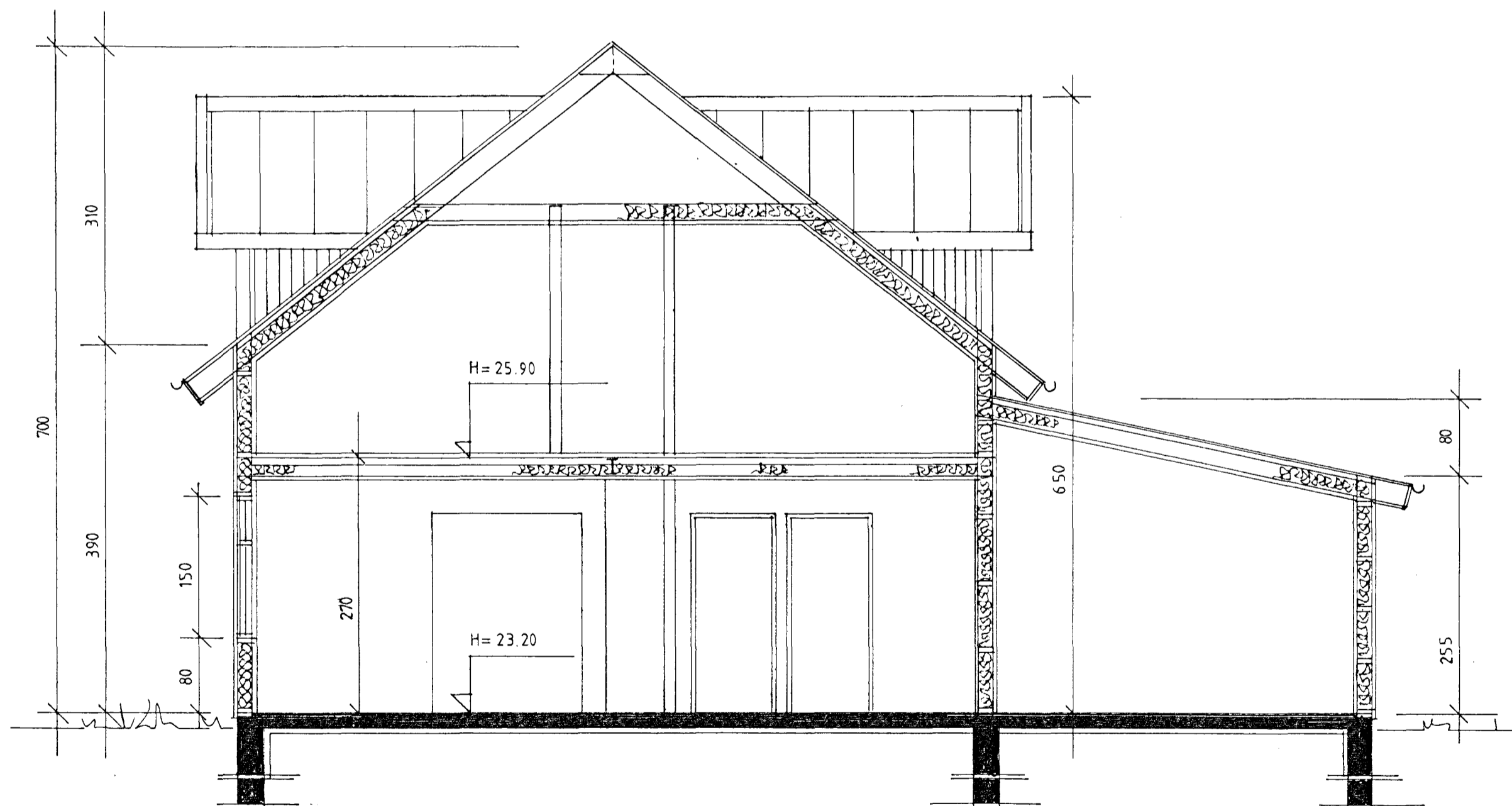
SNID B-B 1:50
