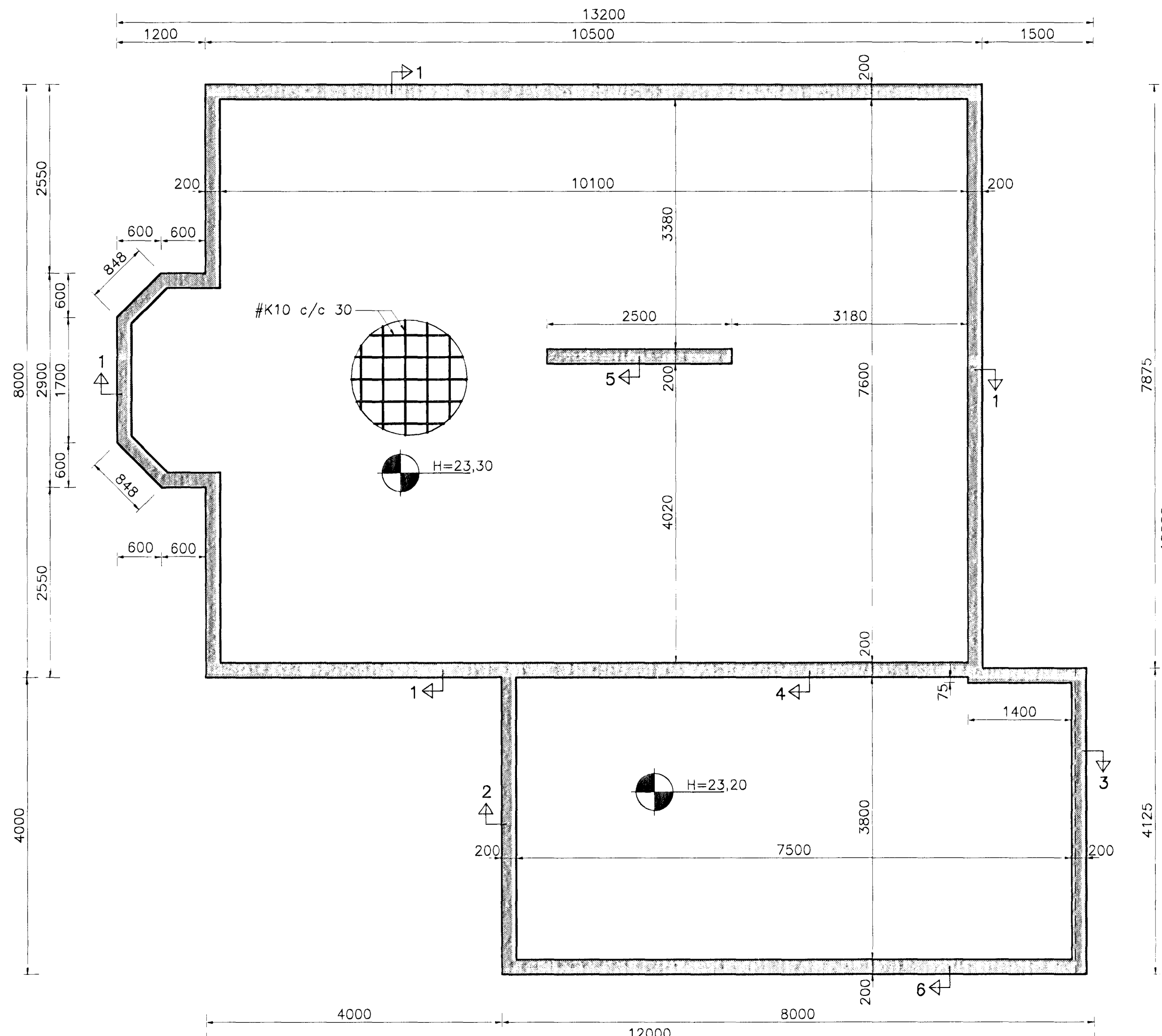
SÖKKLAR GRUNNMYND mkv. 1:50
