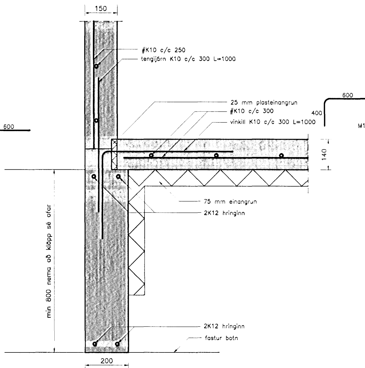
Snið 3-3 Mkv. 1 : 10
