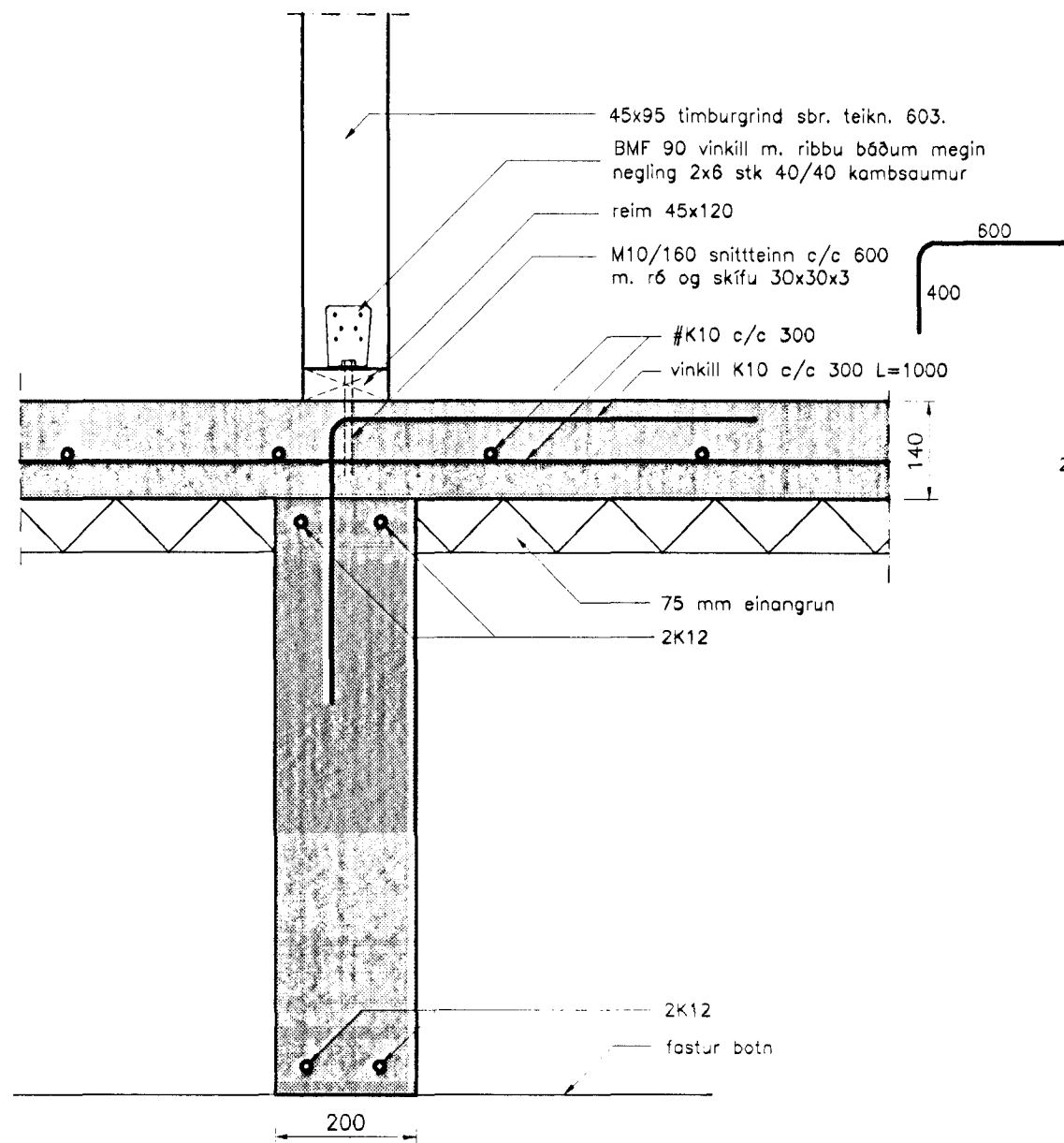
Snið 5-5 Mkv. 1 : 10
