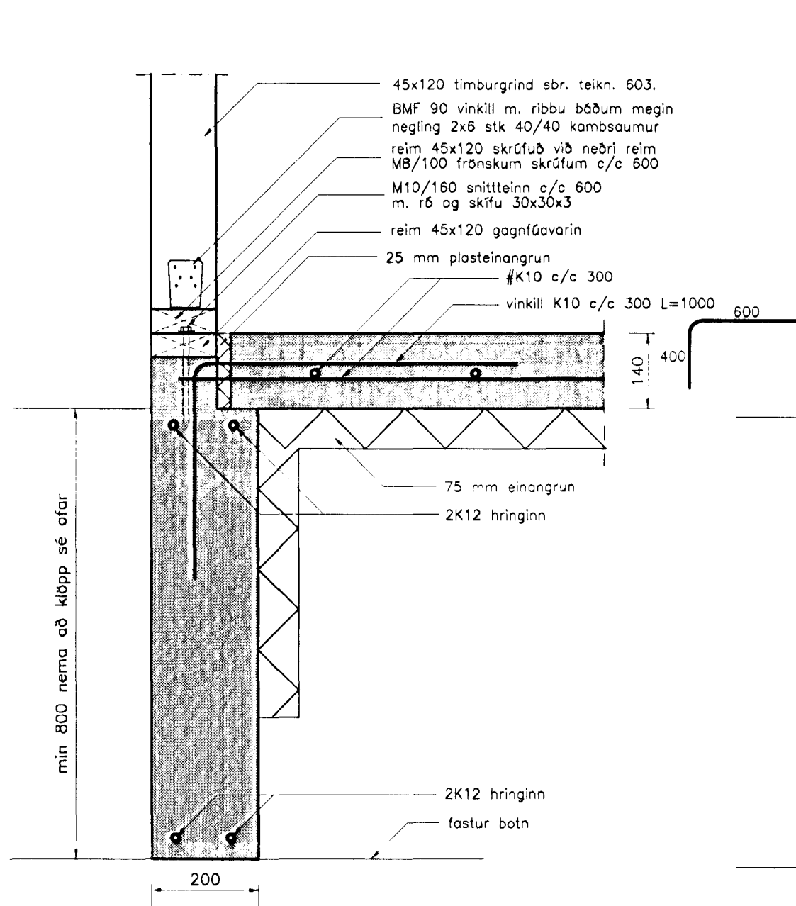
Snið 1-1 Mkv. 1 : 10
