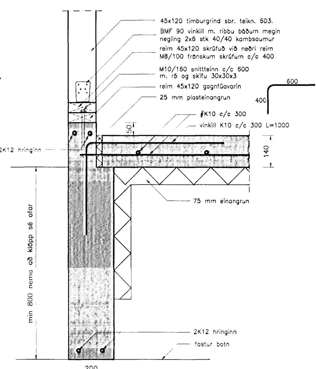
Snið 6-6 Mkv. 1 : 10
