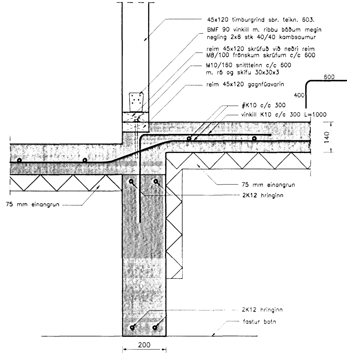
Snið 4-4 Mkv. 1 : 10
