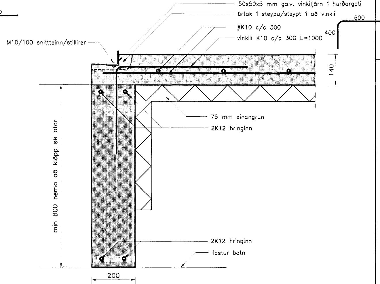
Snið 2-2 Mkv. 1 : 10
