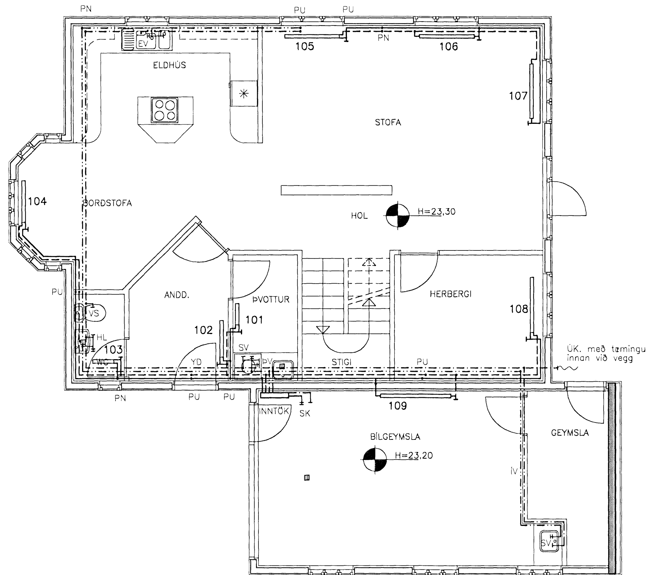
NEYSLUVATNS- OG HITLAGNIR GRUNNMYND NEDRI HÆÐAR mkv. 1:50
