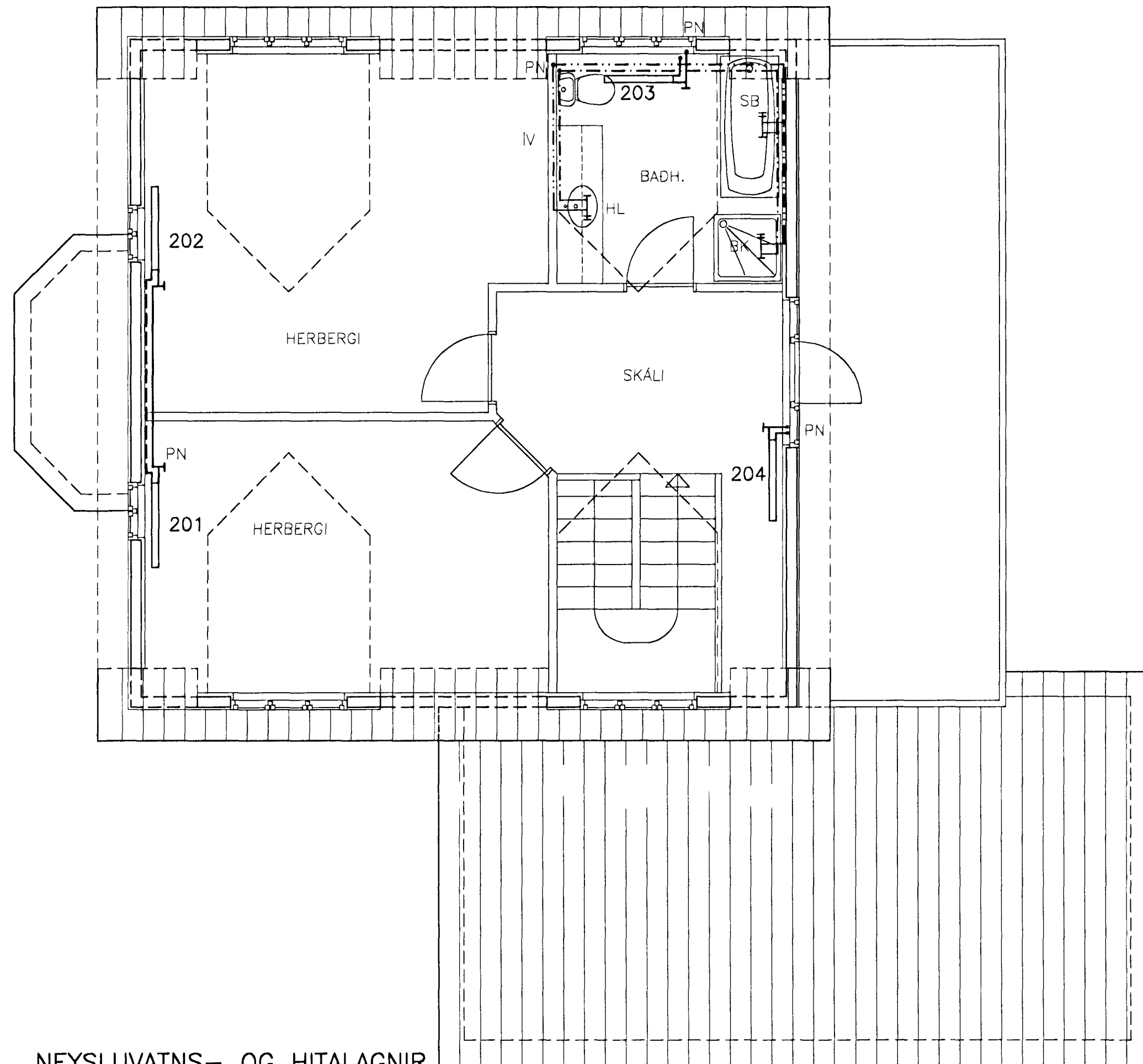
NEYSLUVATNS- OG HITALAGNIR GRUNNMYND EFRI HÆÐAR mkv. 1:50
