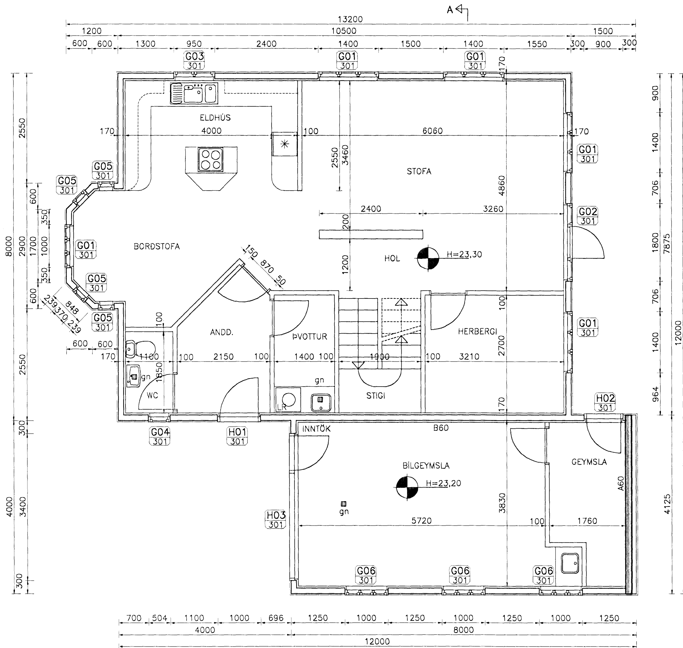
GRUNNMYND NEDRI HÆÐAR mkv. 1:50
