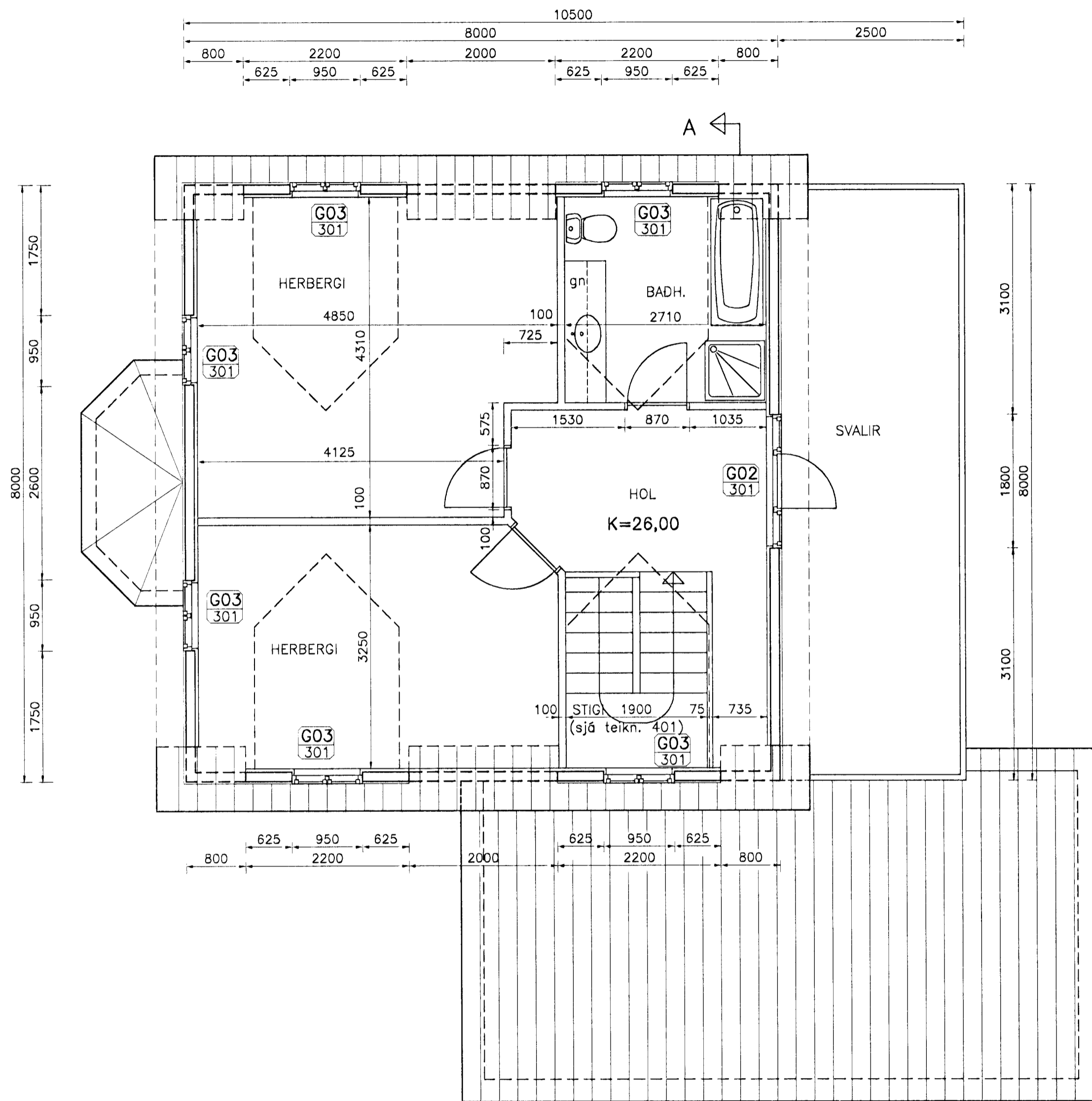
GRUNNMYND EFRI HÆÐAR mkv. 1:50
