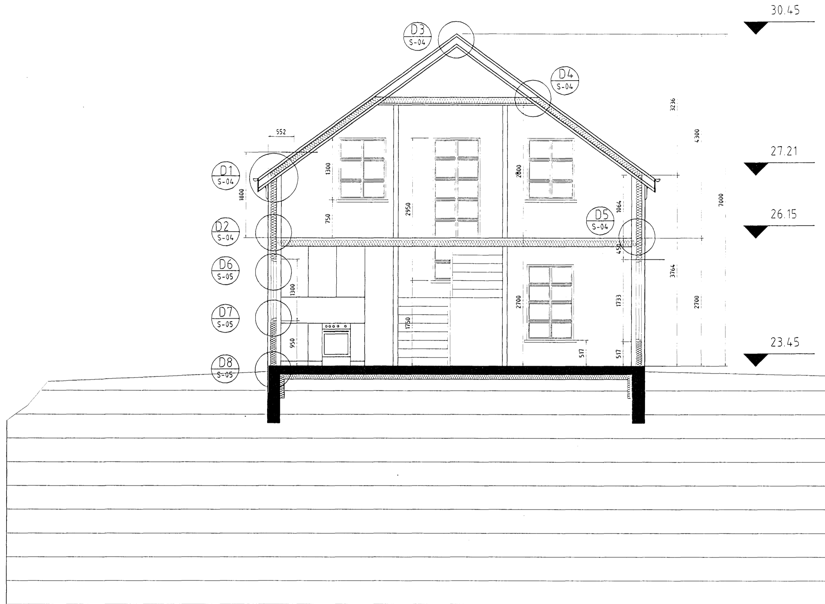
SNEIÐING A-A
