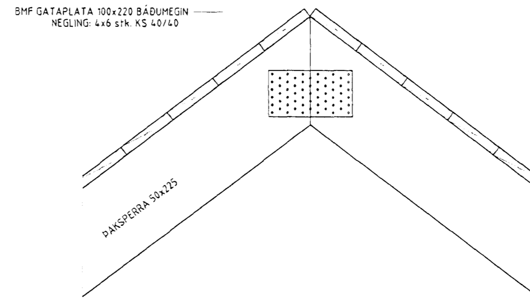
DEILI 5 mkv. 1:10
