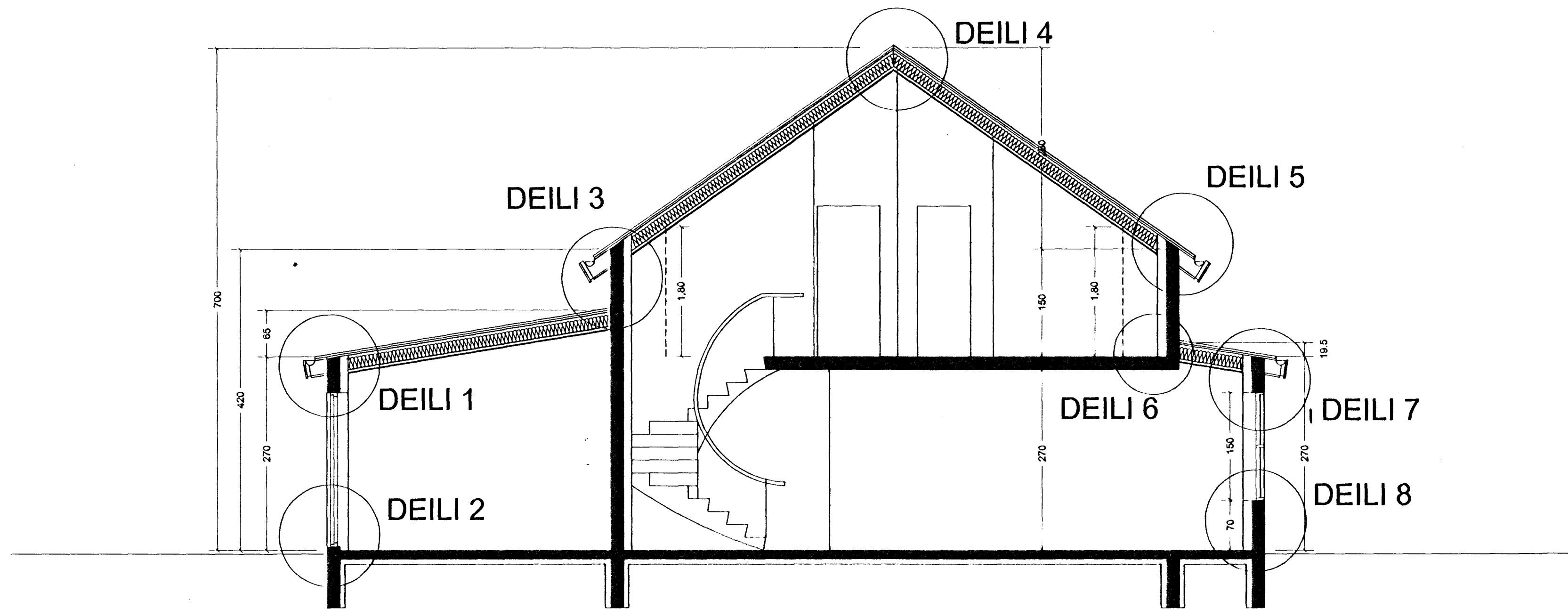
SKURÐUR A-A
