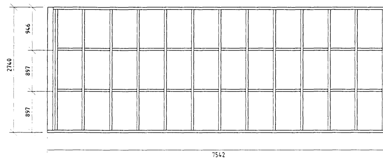
VEGGJAGRIND VESTURHLIÐAR
