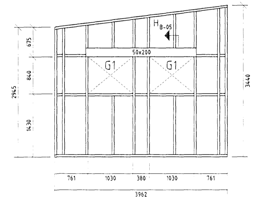
VEGGJAGRIND SUÐURHLIÐAR
