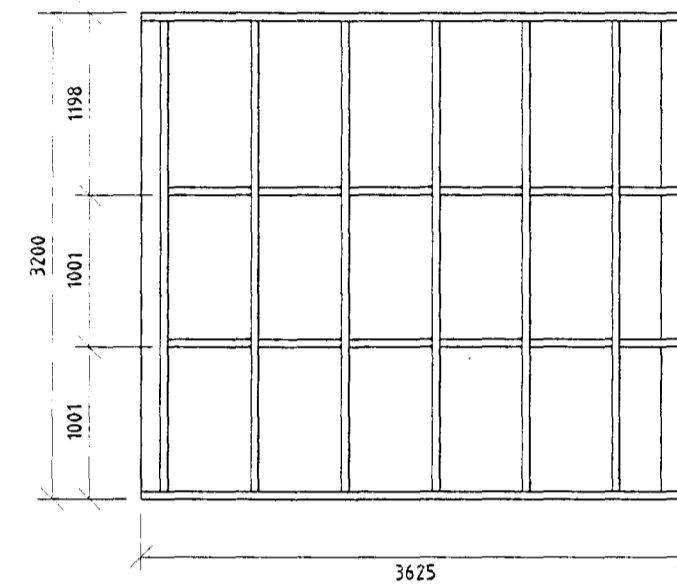
VEGGJAGRIND AUSTURHLIÐAR
