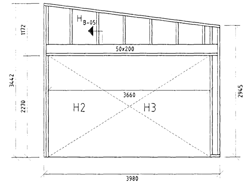
VEGGJAGRIND NORÐURHLIÐAR
