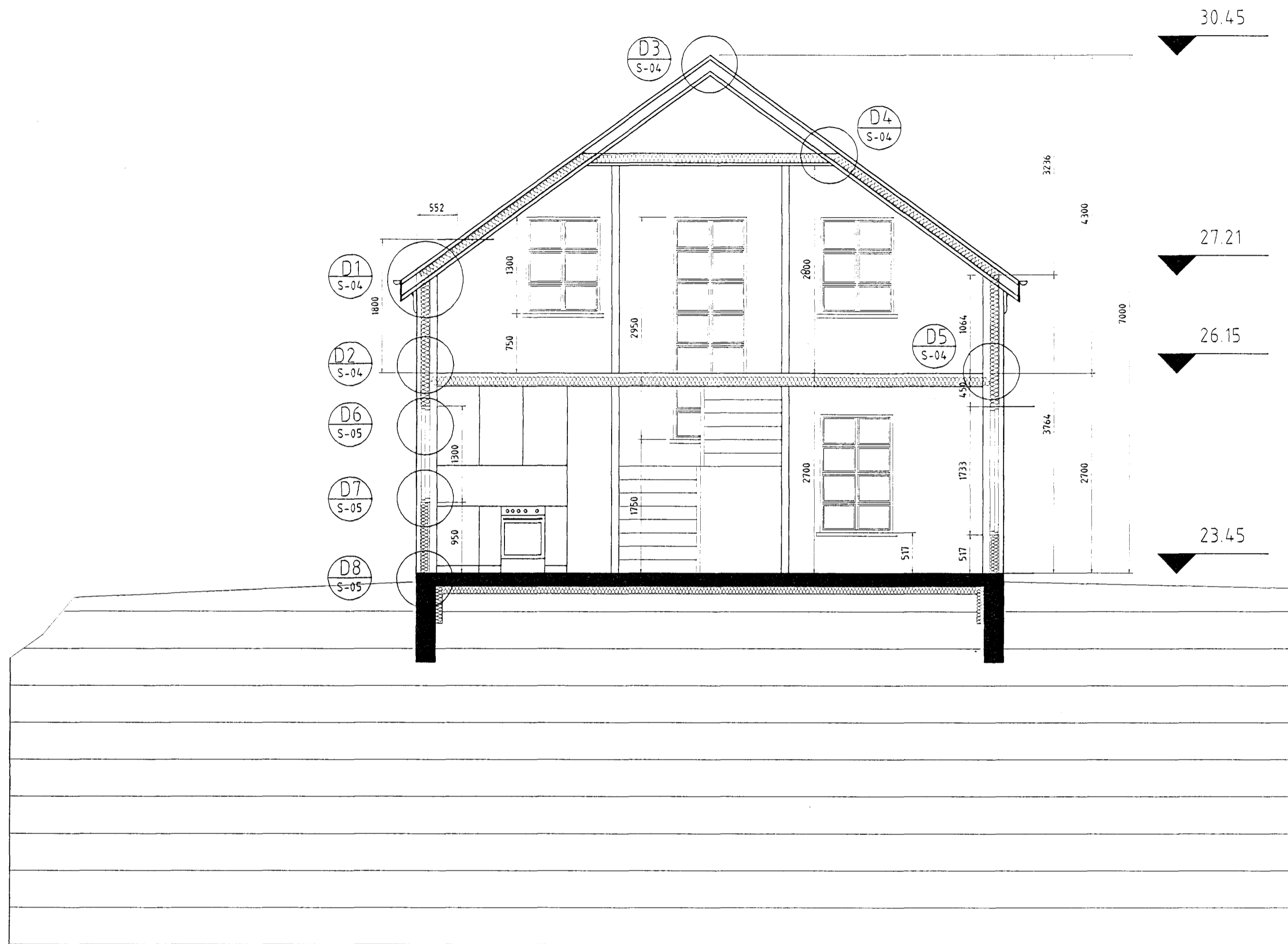
SNEIÐING A-A
