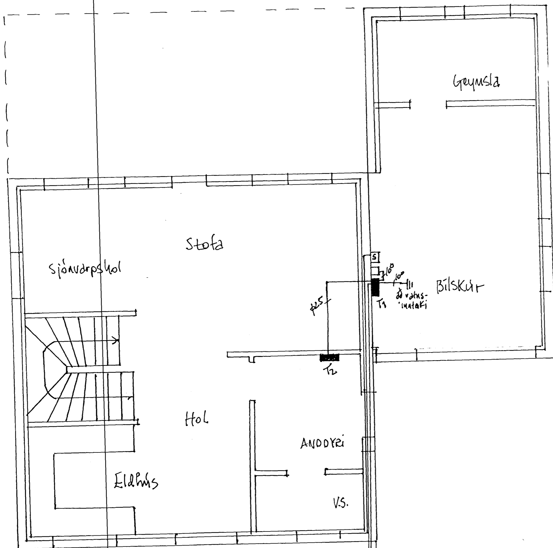
GRUNNMYPND 1. Hæðar 1:50
