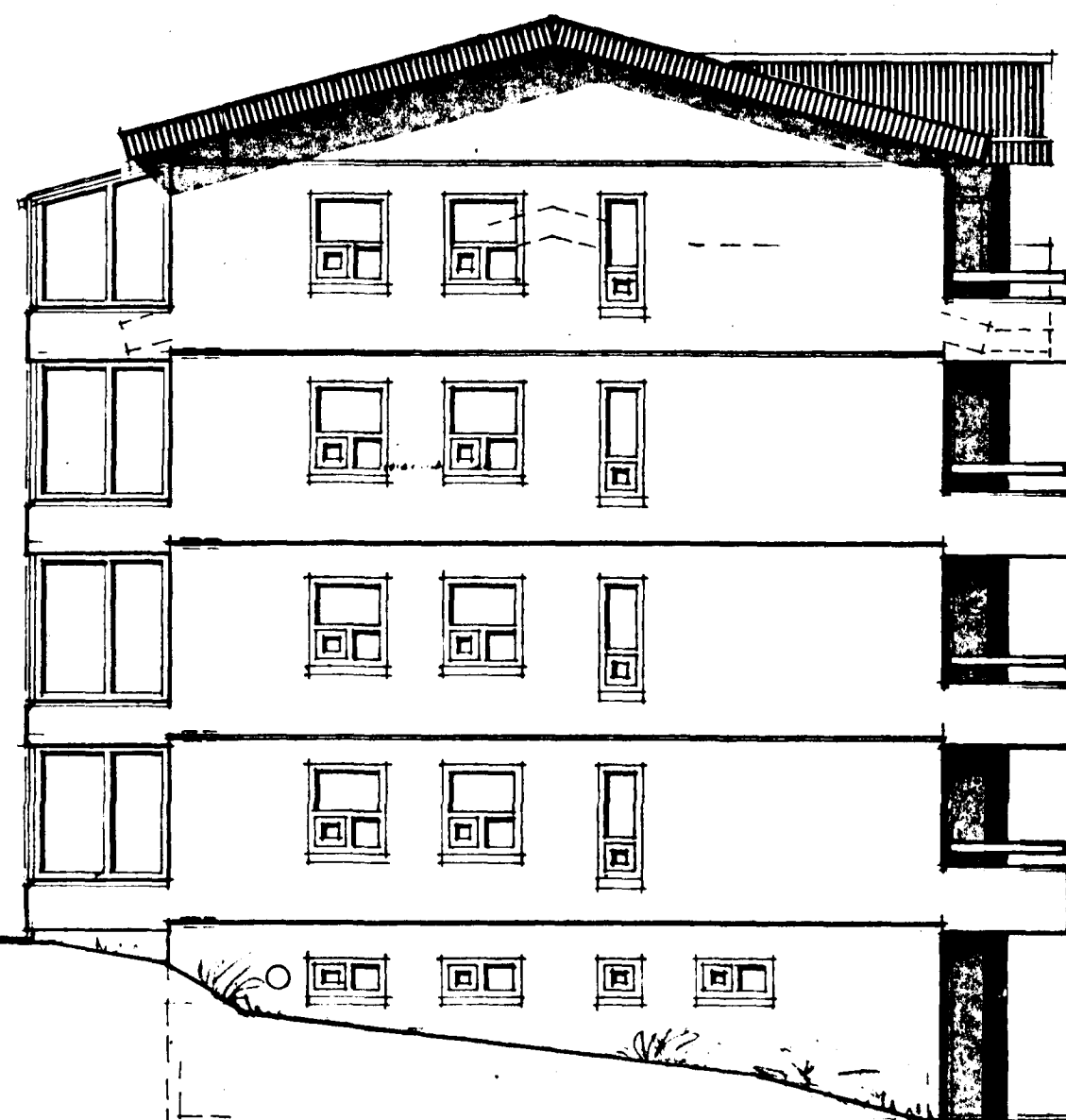
AUSTURHLIÐ
