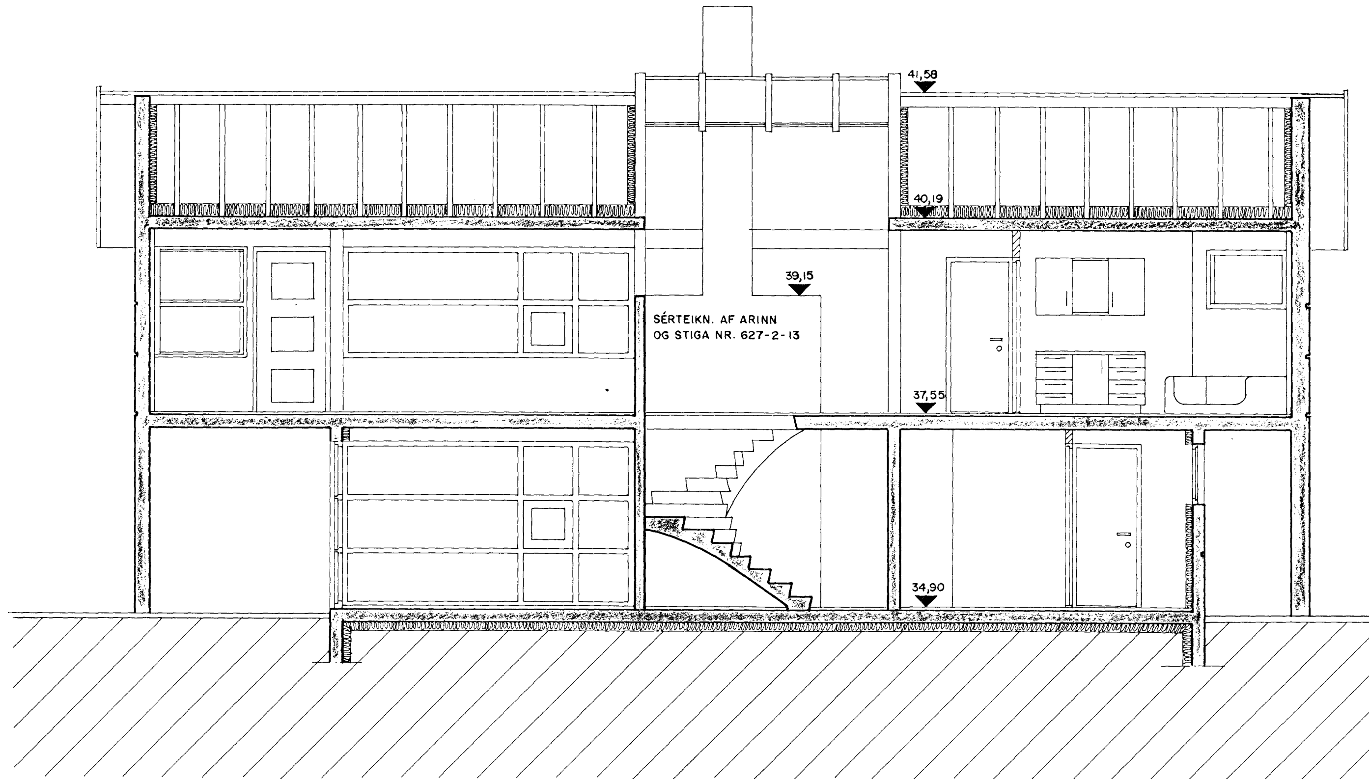
SNEIÐING 13-13
