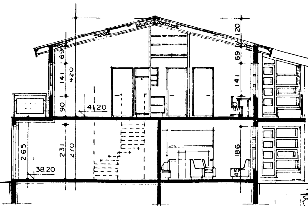
SNEIÐING A-A
