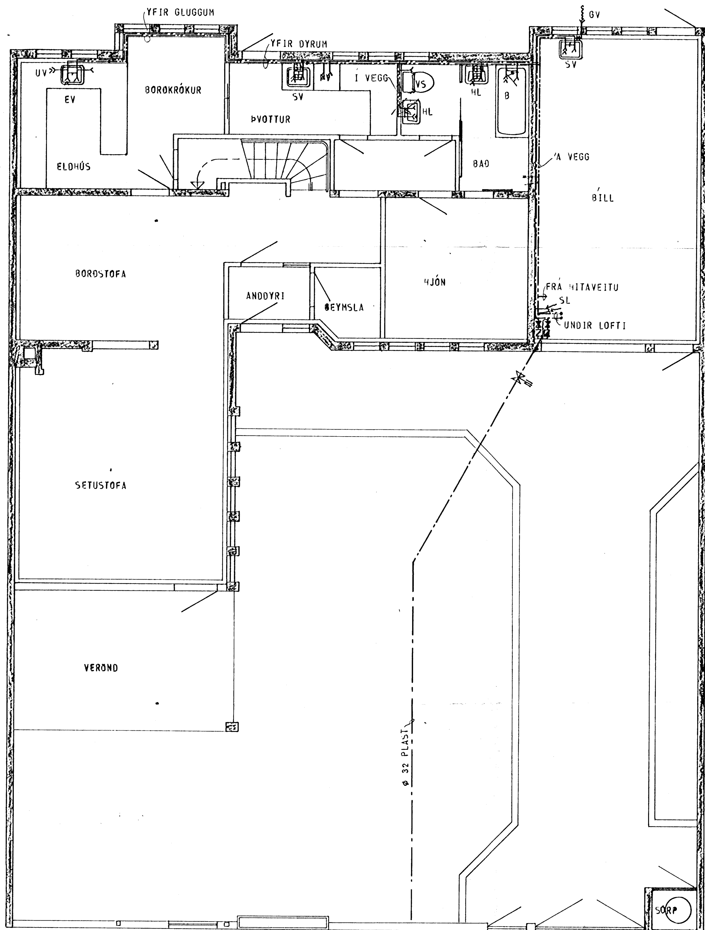
GRUNNMYND - HÆÐAR 1:50
