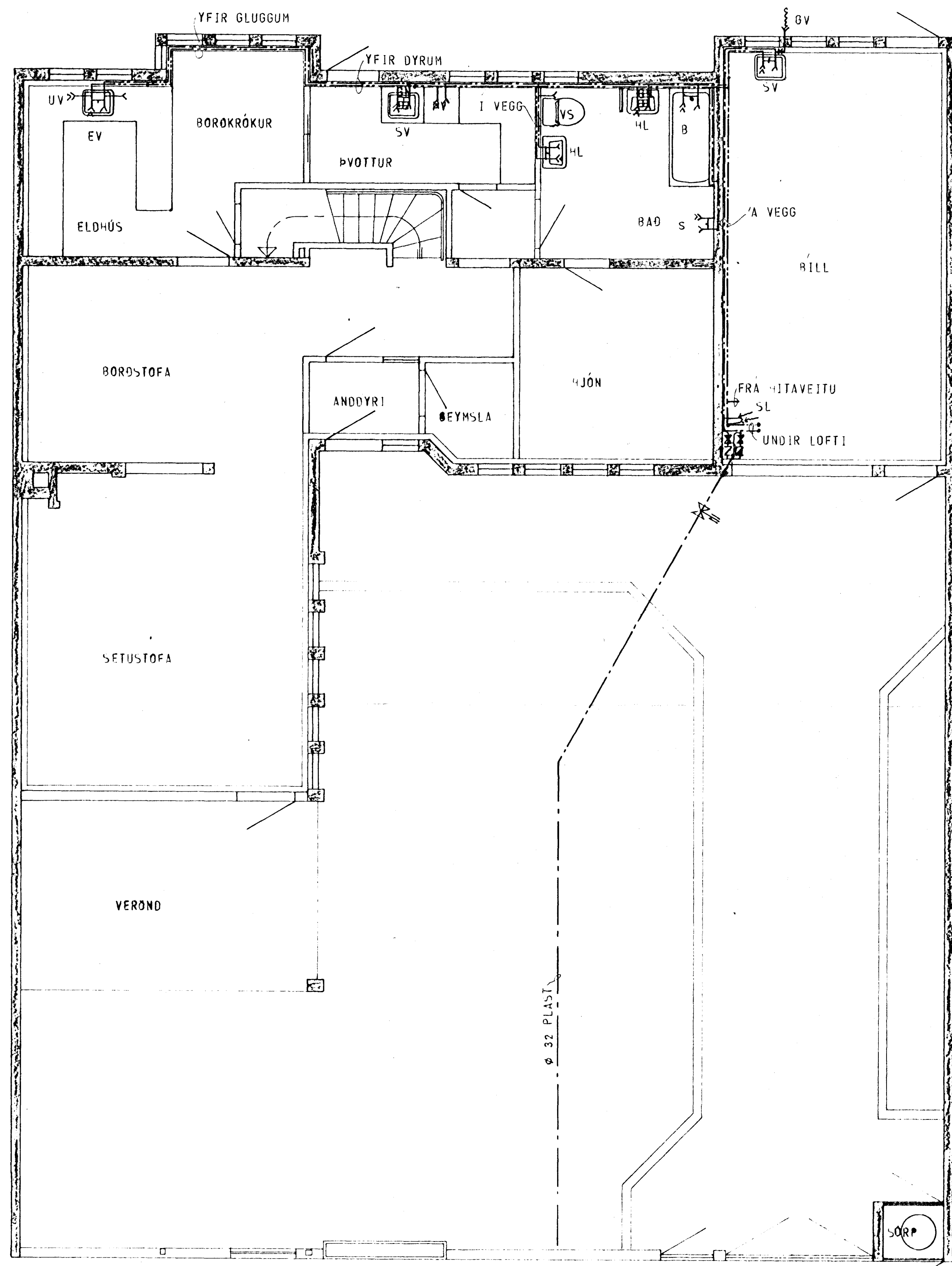
GRUNNMYND - HÆÐAR 1:50
