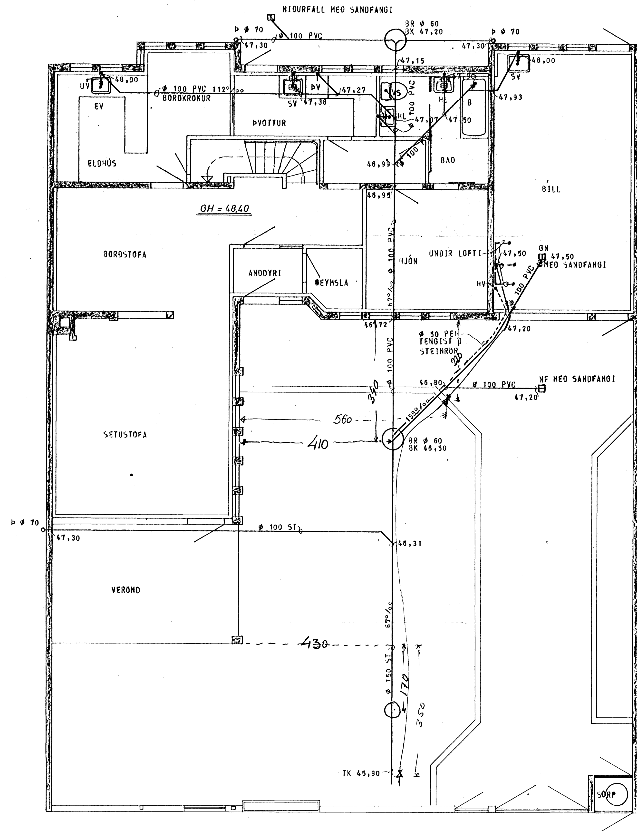
GRUNNMYND - HÆÐAR 1:50
