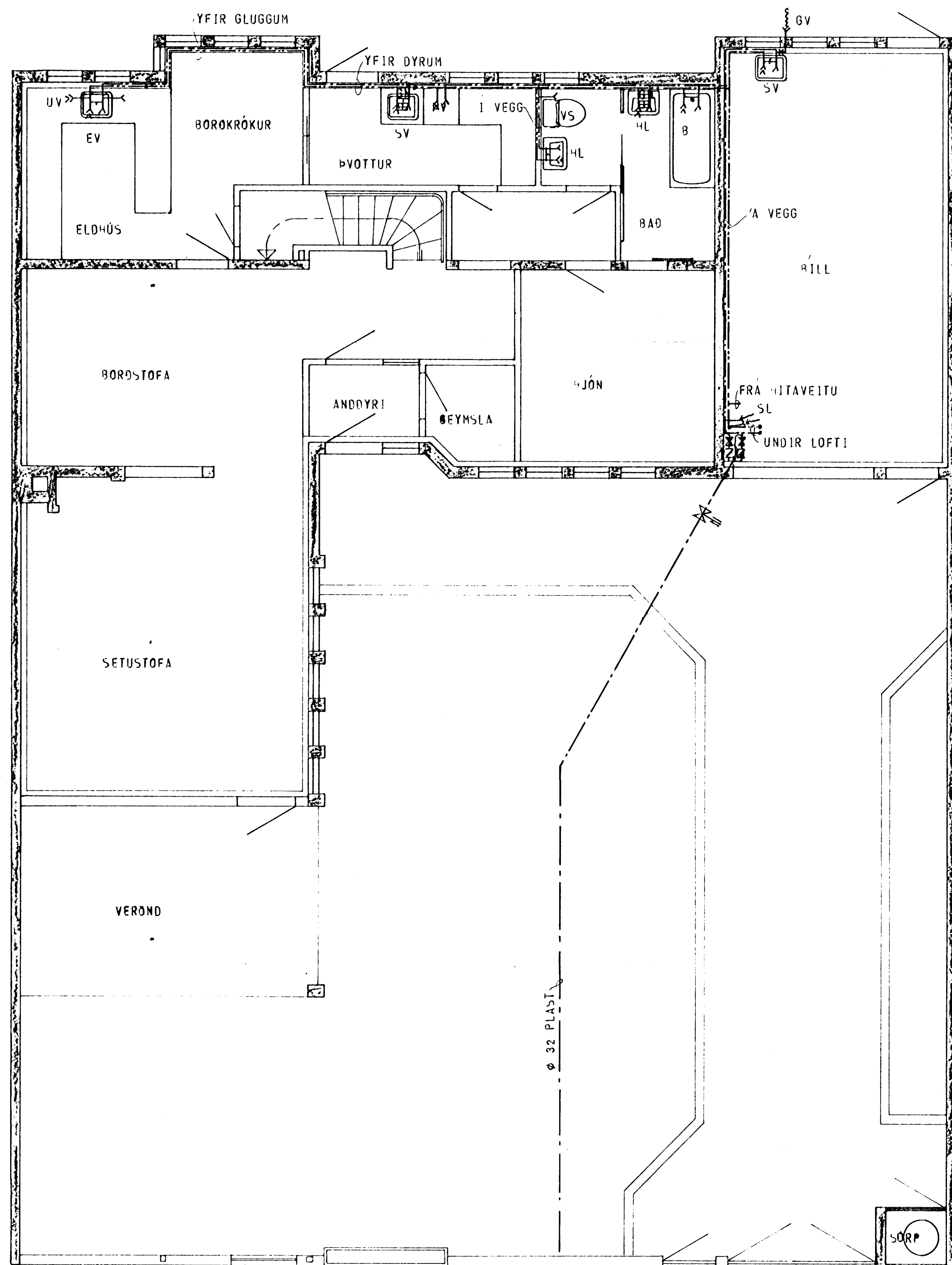
GRUNNMYND - HÆÐAR 1:50
