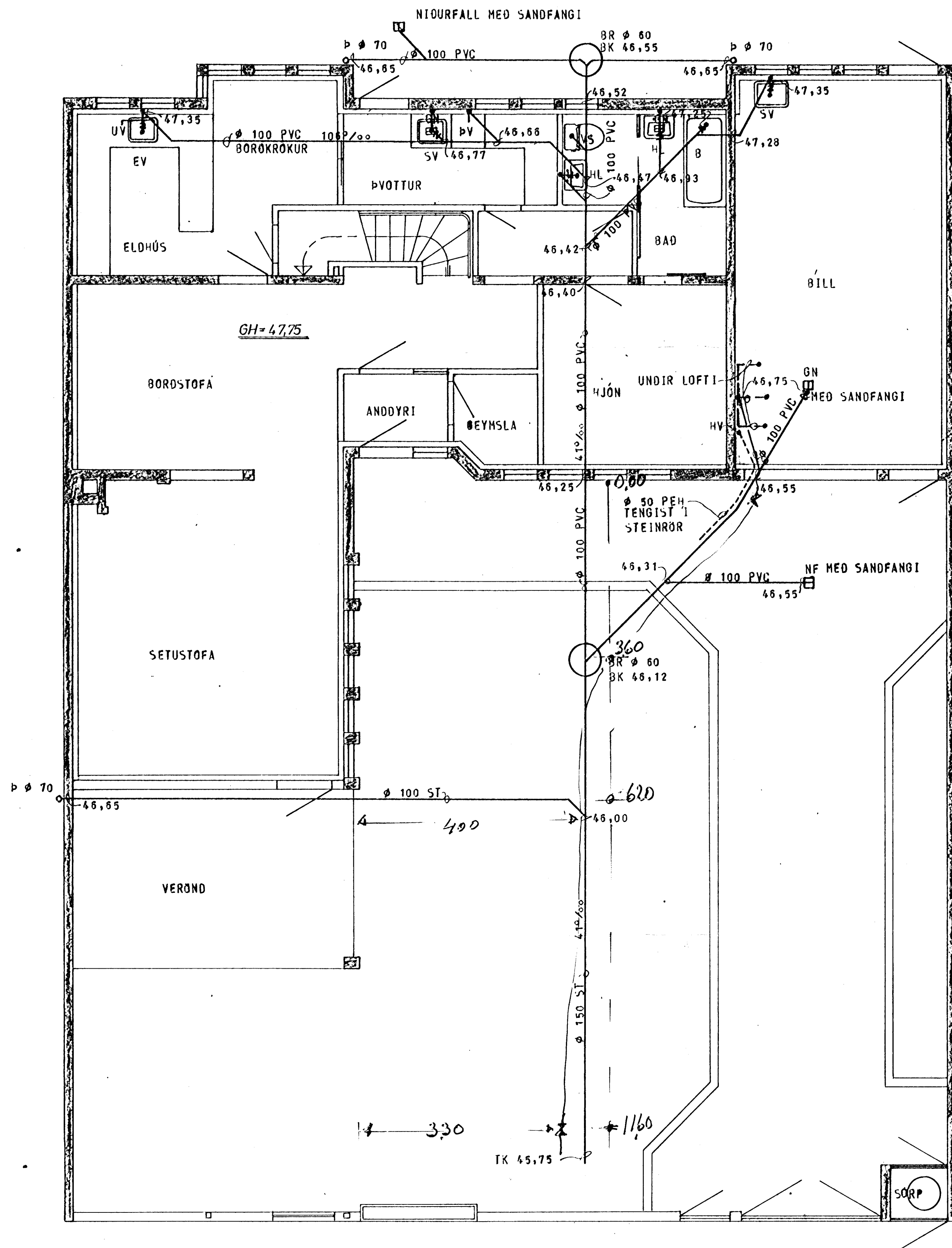
GRUNNMYND - HÆÐAR 1:50
