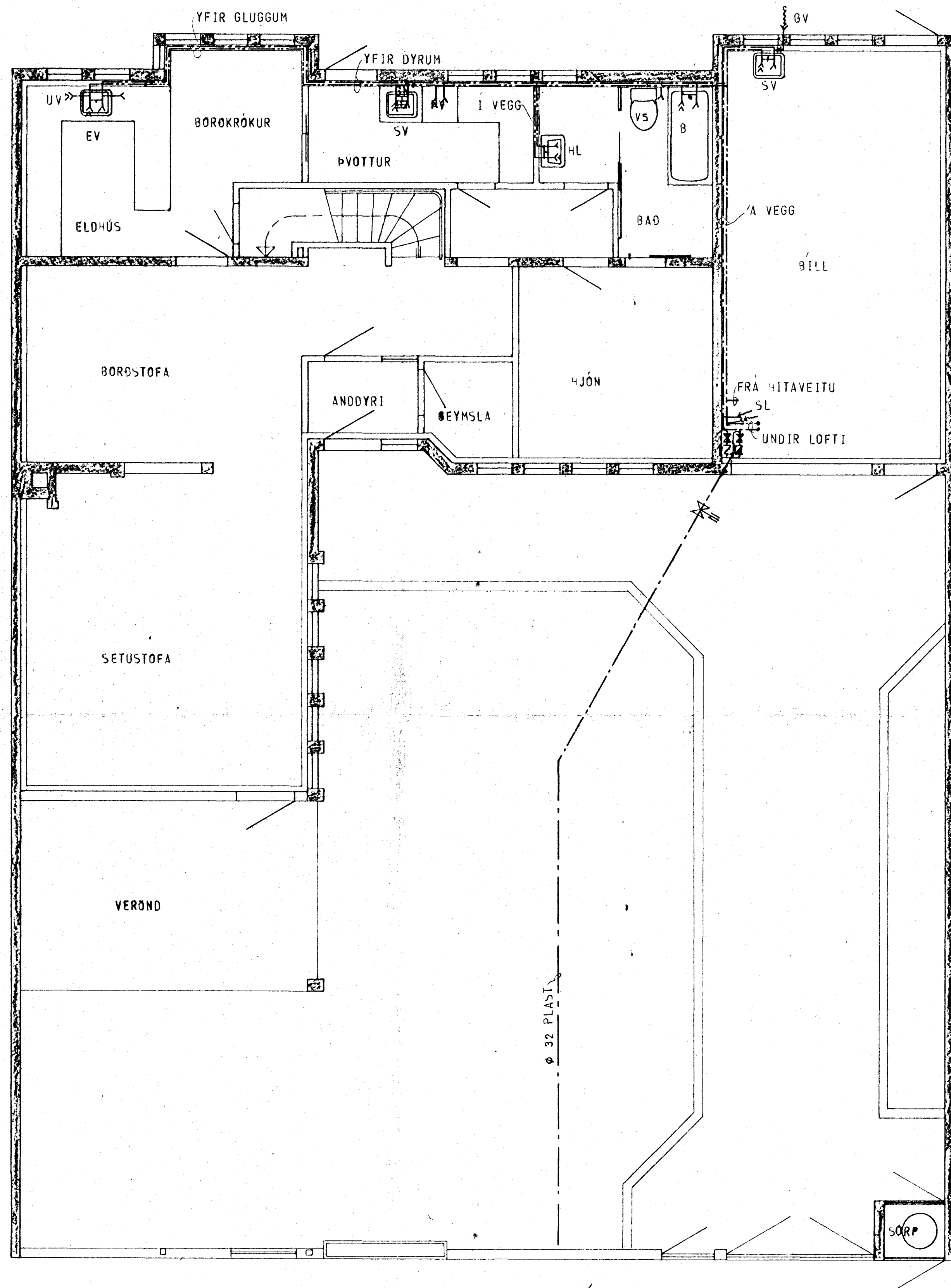
GRUNNMYND - HÆÐAR 1:50
