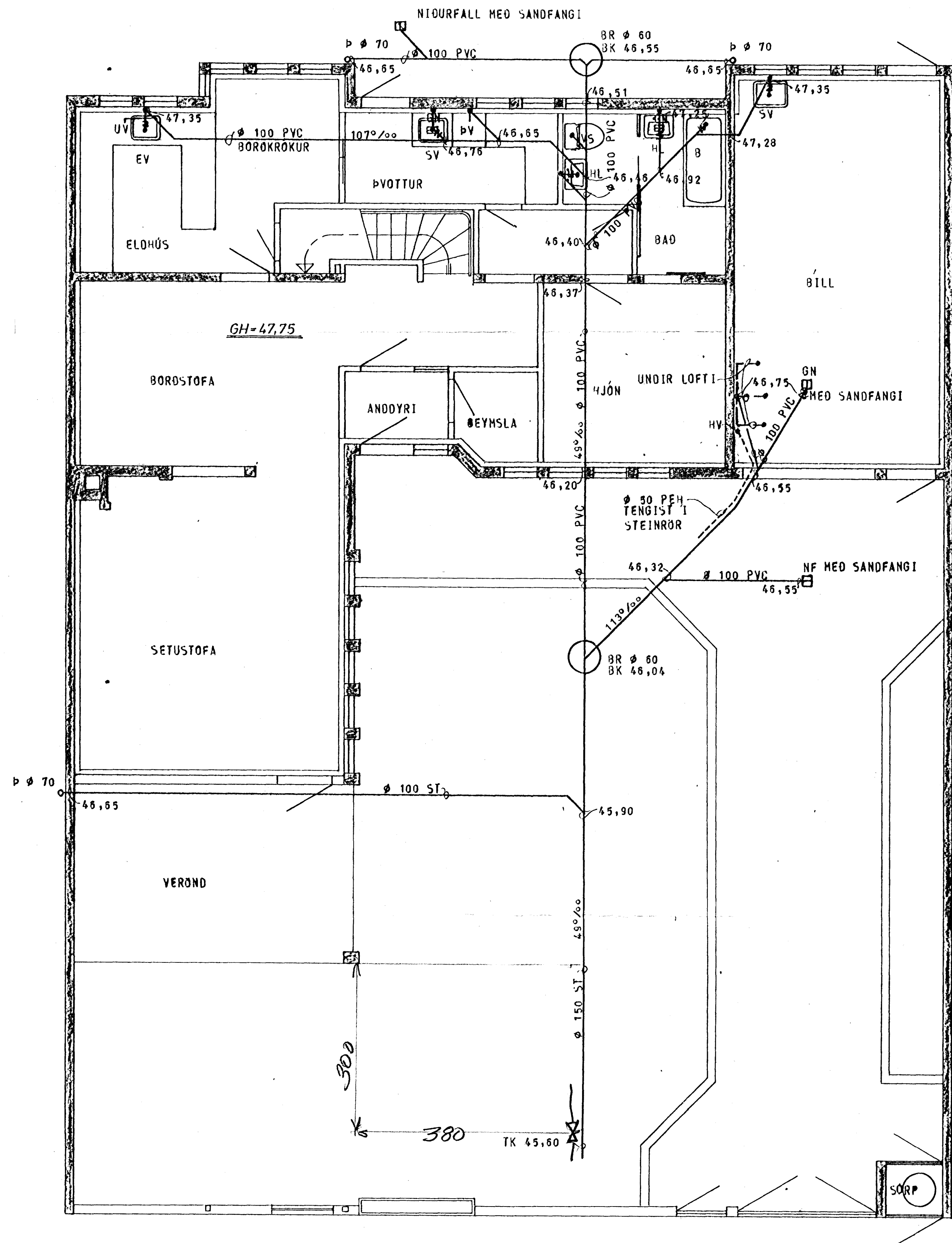
GRUNNMYND - HÆÐAR 1:50
