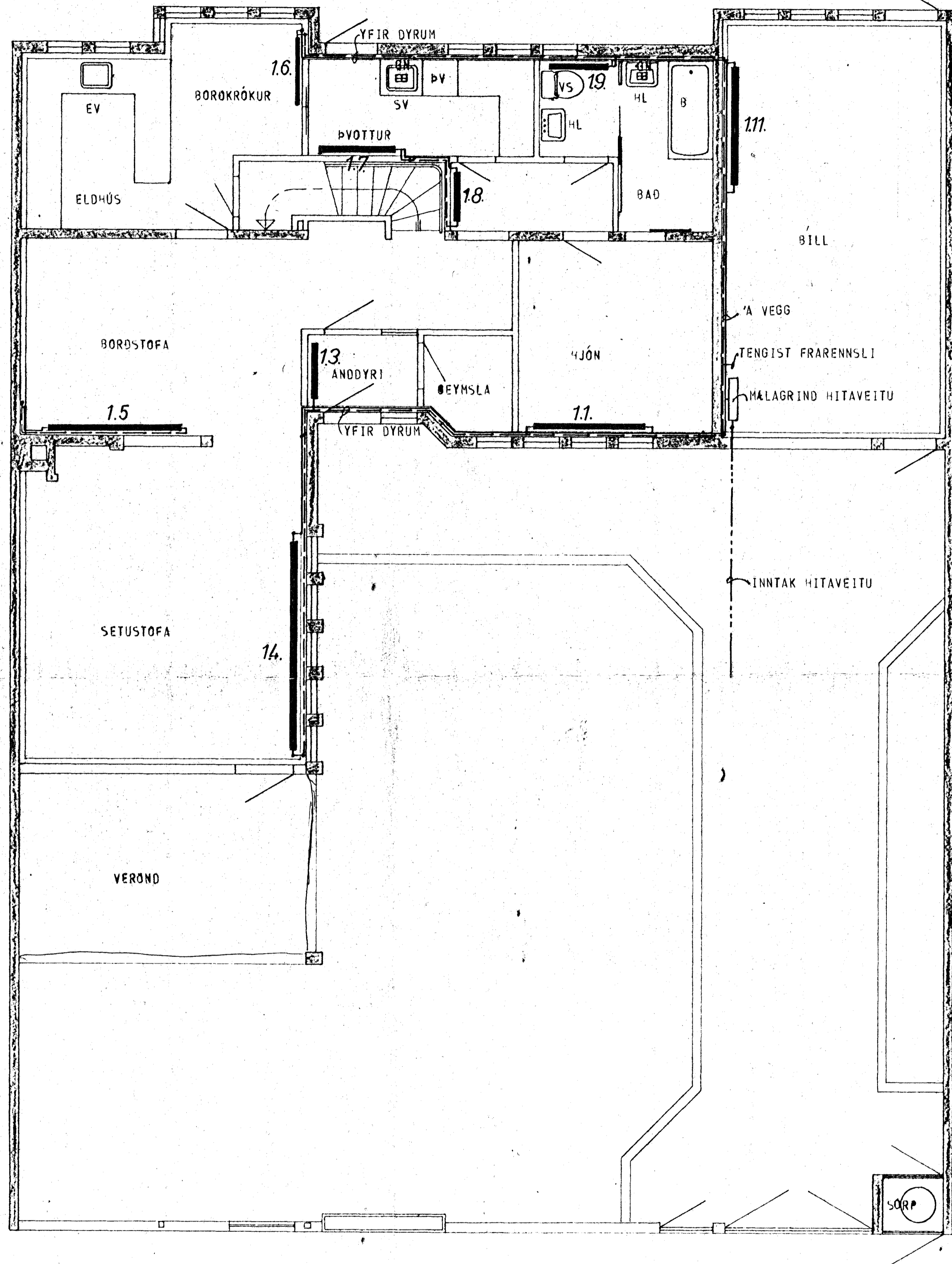
GRUNNMYND - HÆÐAR 1:50
