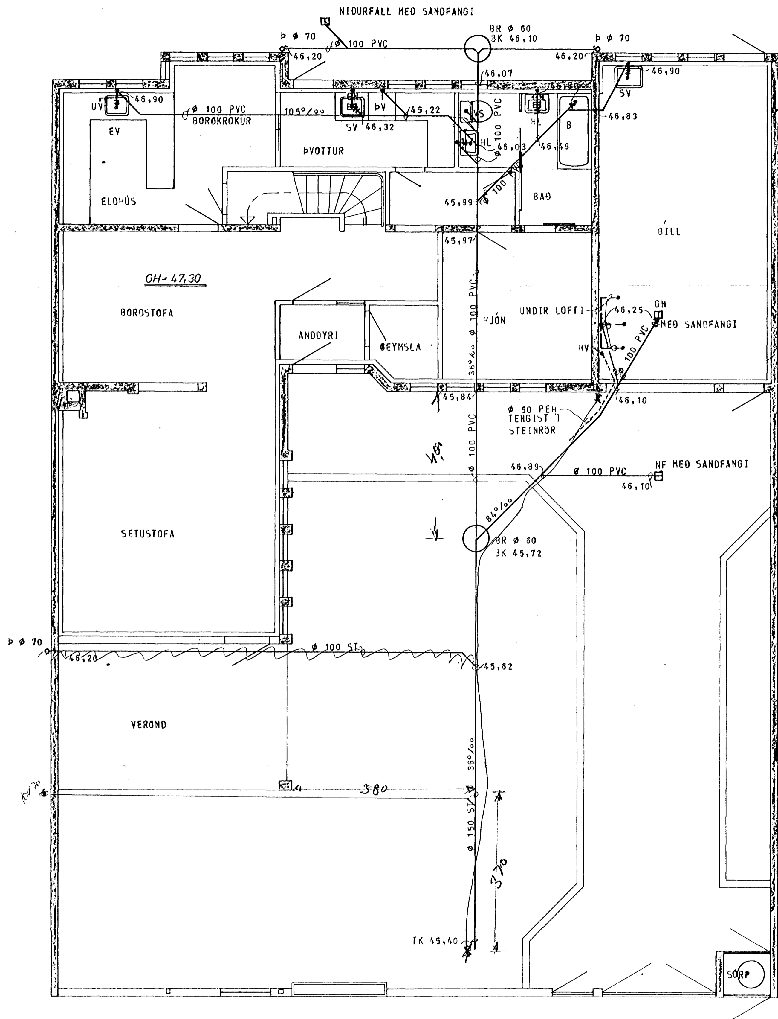
GRUNNMYND - HÆÐAR 1:50
