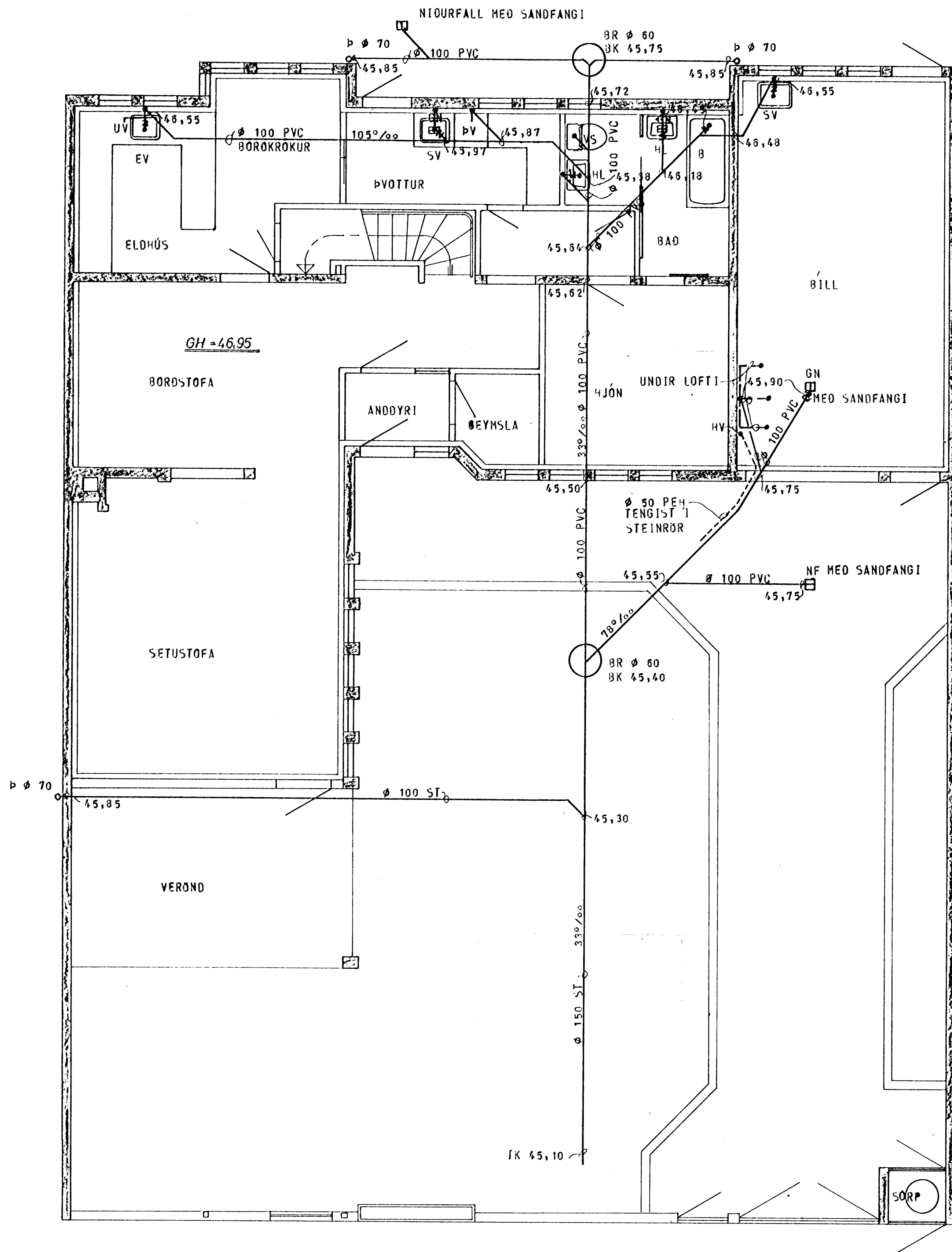
GRUNNMYND - HÆÐAR 1:50
