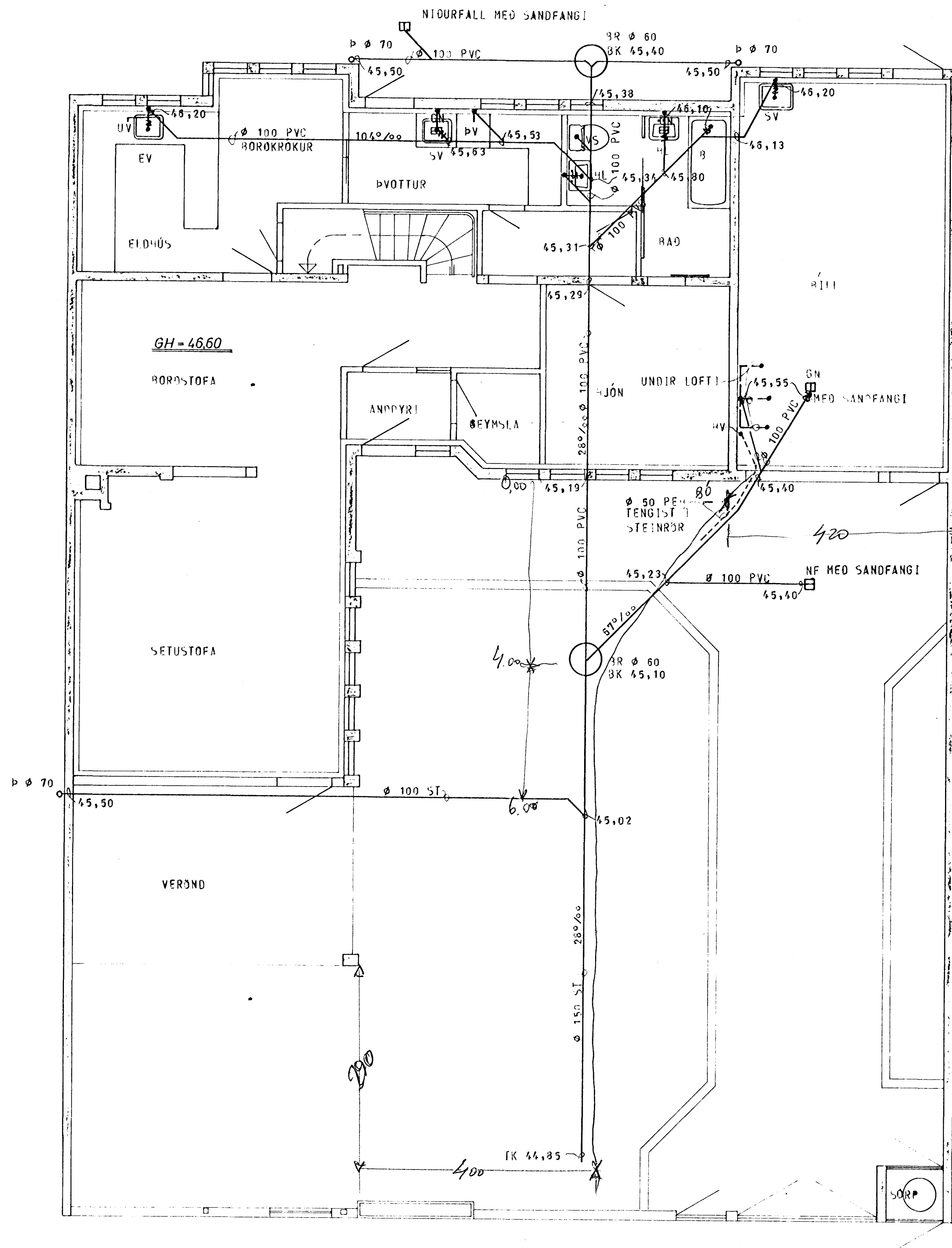
GRUNNMYND - HÆÐAR 1:50
