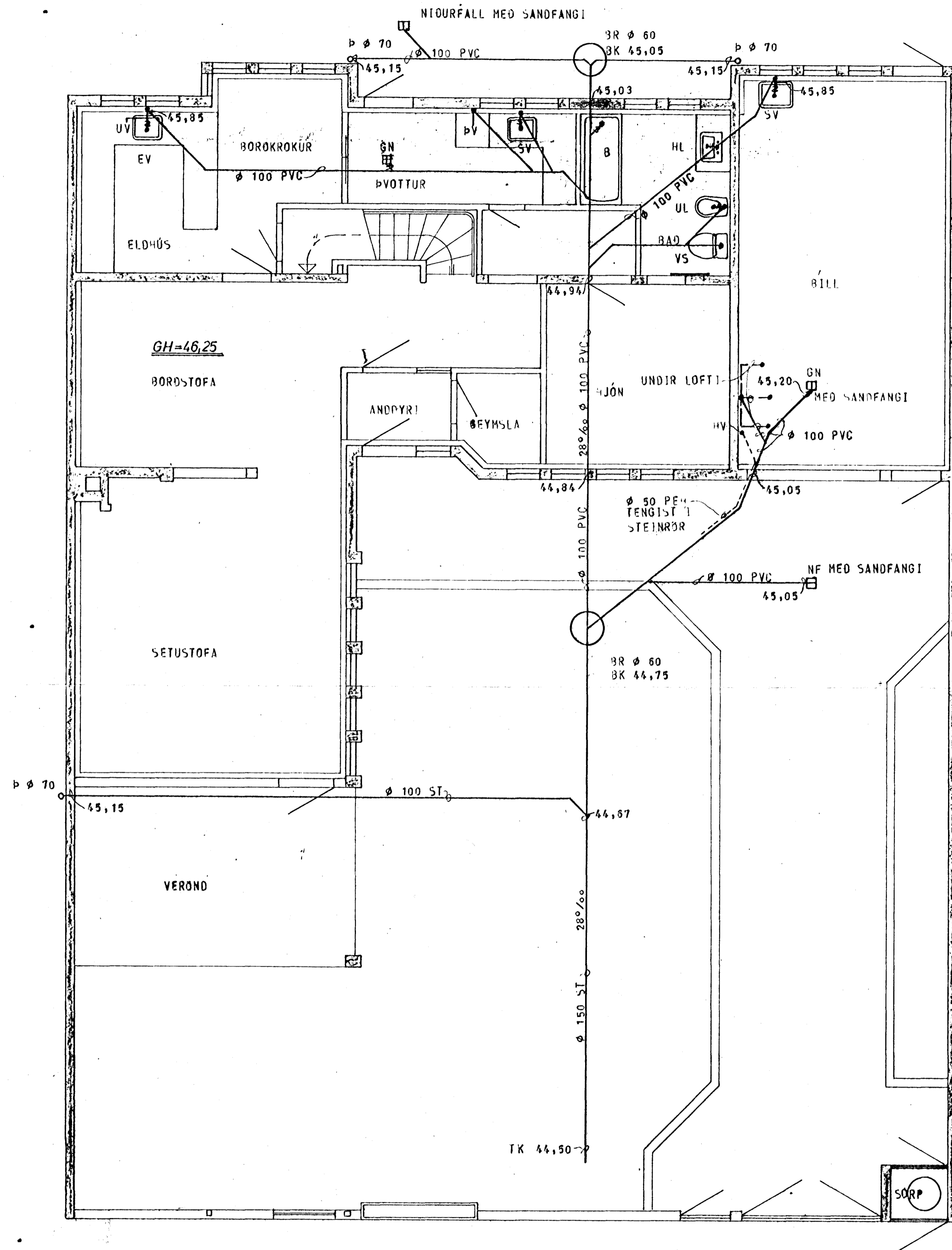
GRUNNMYND - HÆÐAR 1:50
