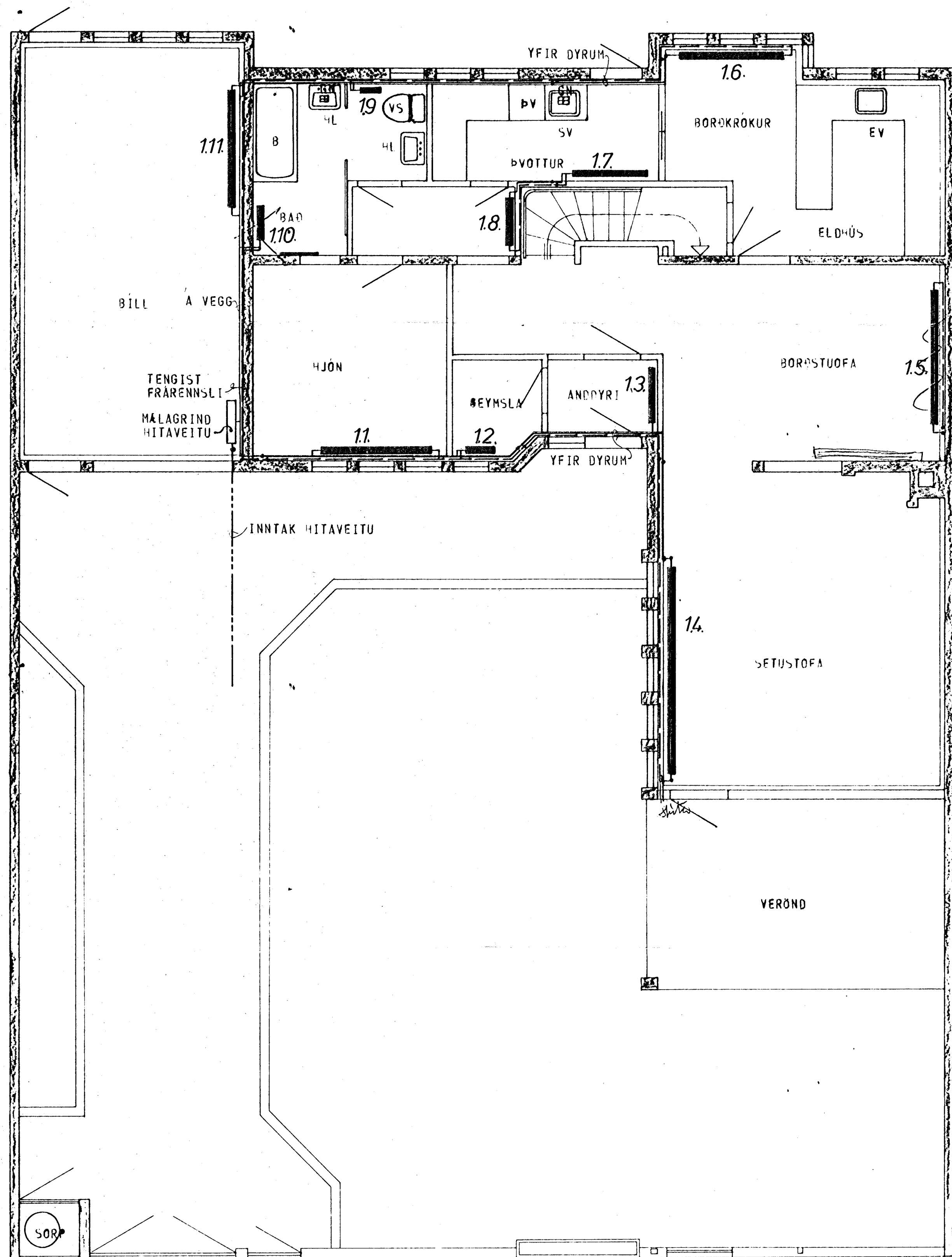
GRUNNMYND - HÆÐAR 1:50
