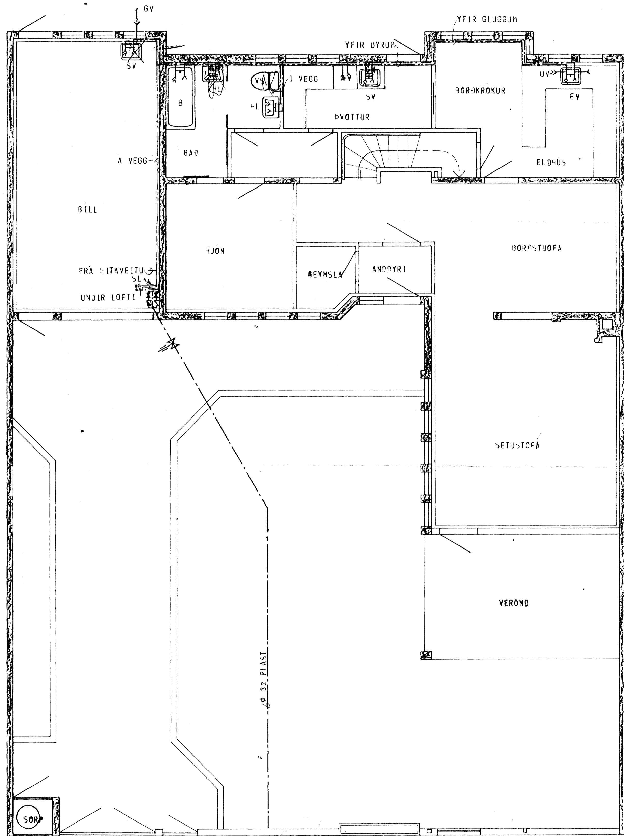
GRUNNMYND - HÆÐAR 1:50
