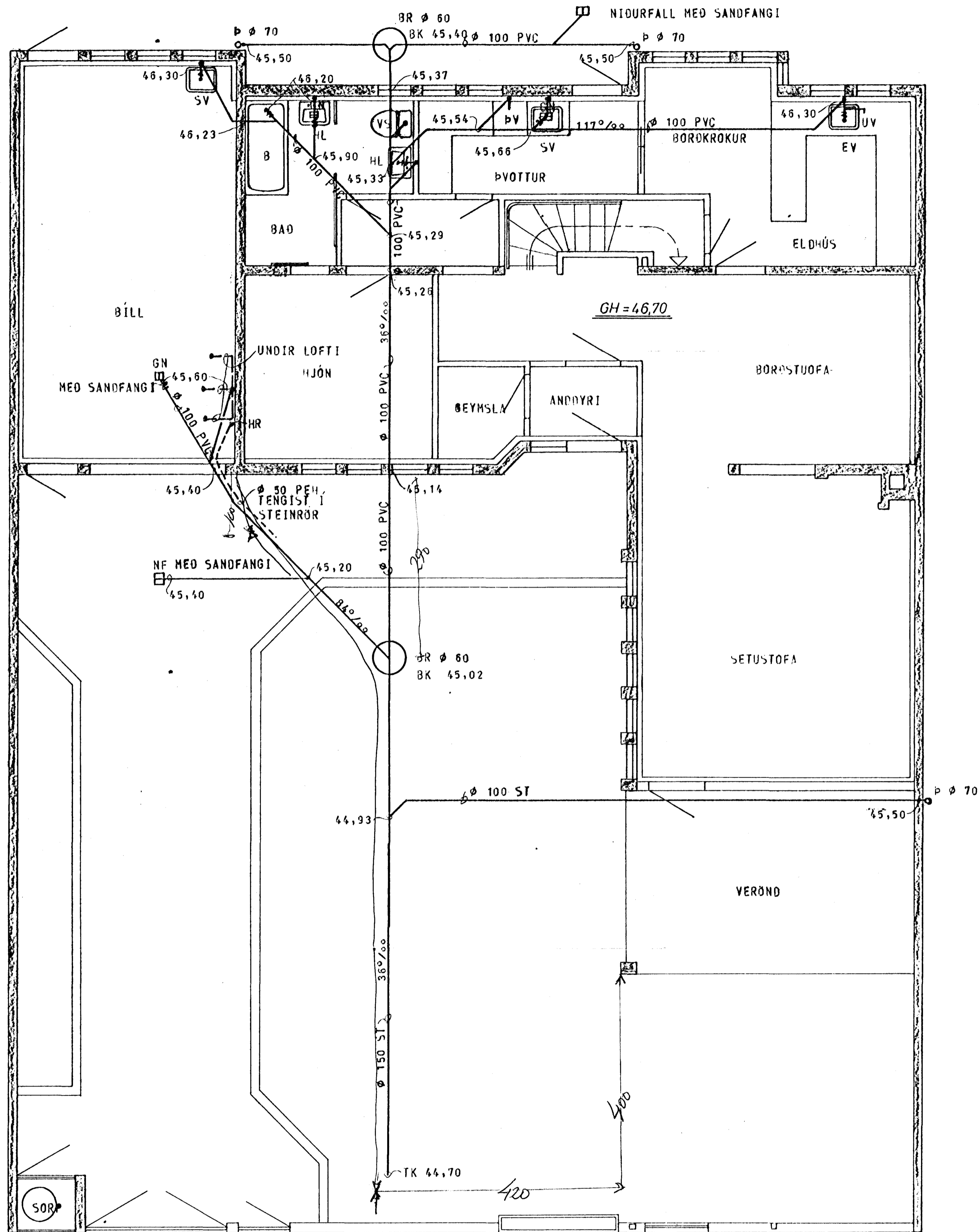
GRUNNMYND - HÆÐAR 1:50
