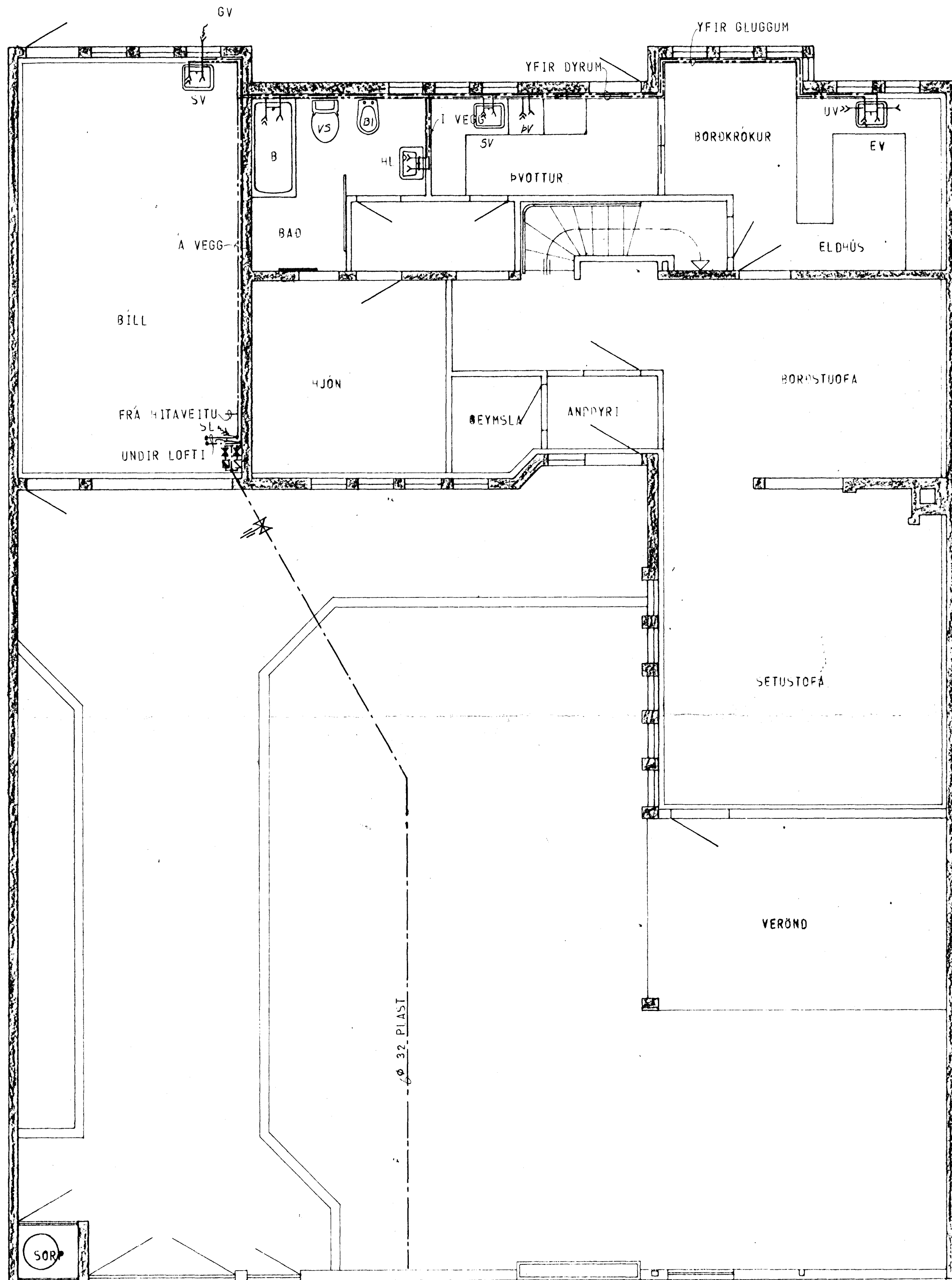
GRUNNMYND - HÆÐAR 1:50
