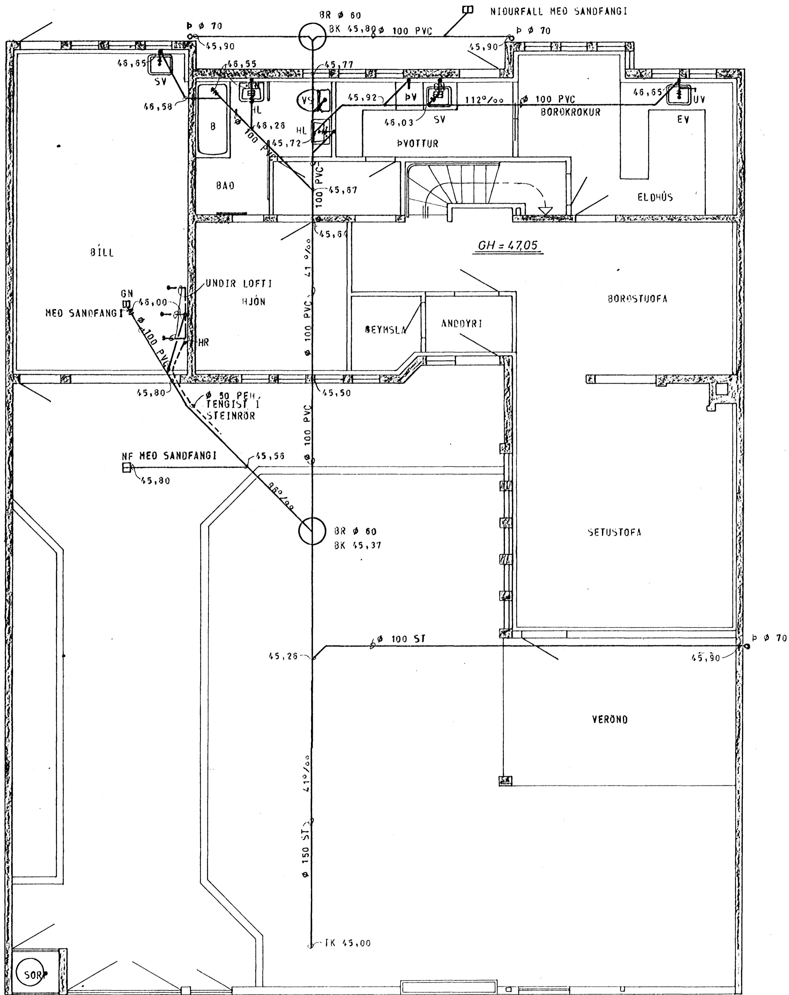
GRUNNMYND - HÆÐAR 1:50
