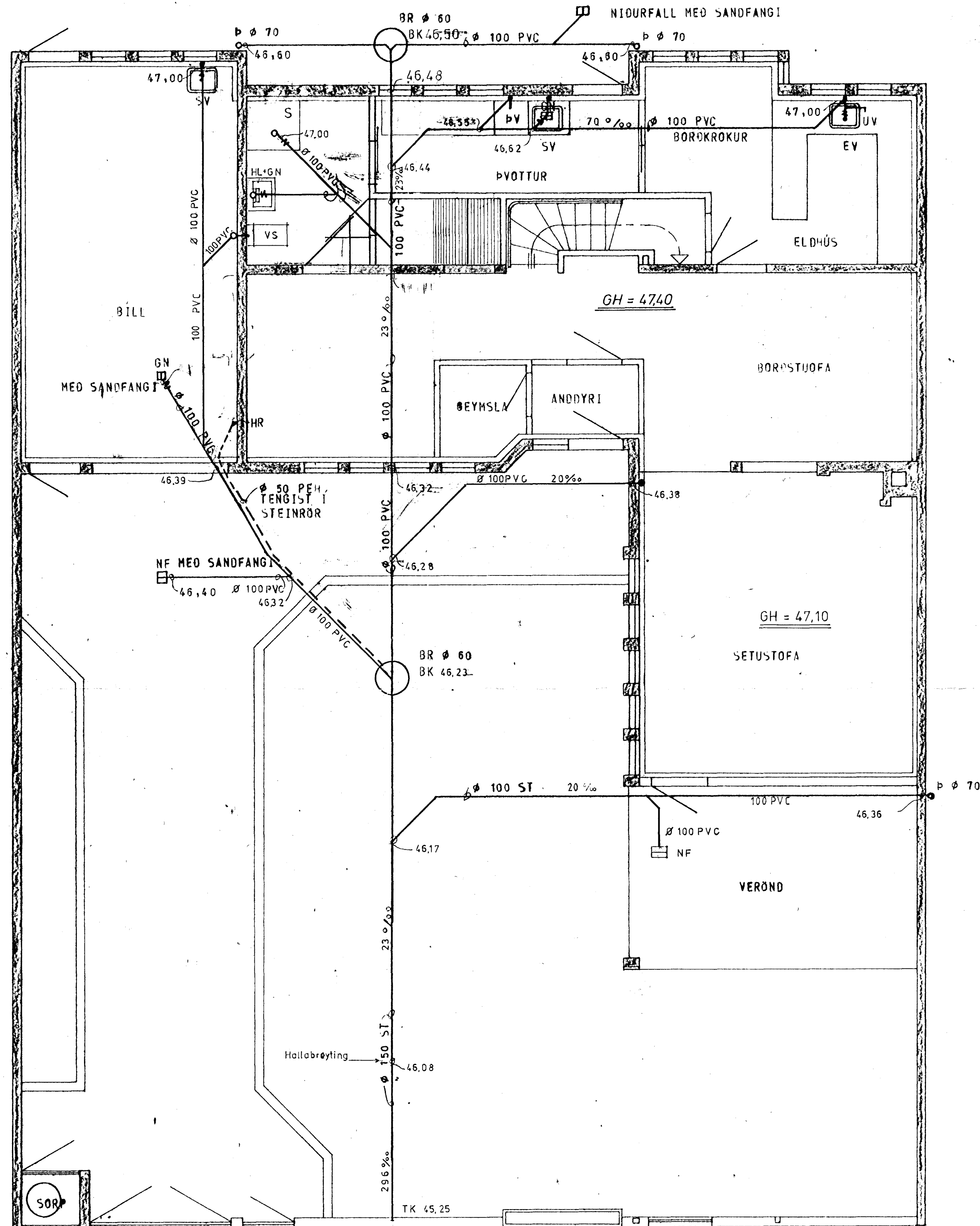
GRUNNMYND - HÆÐAR 1:50
