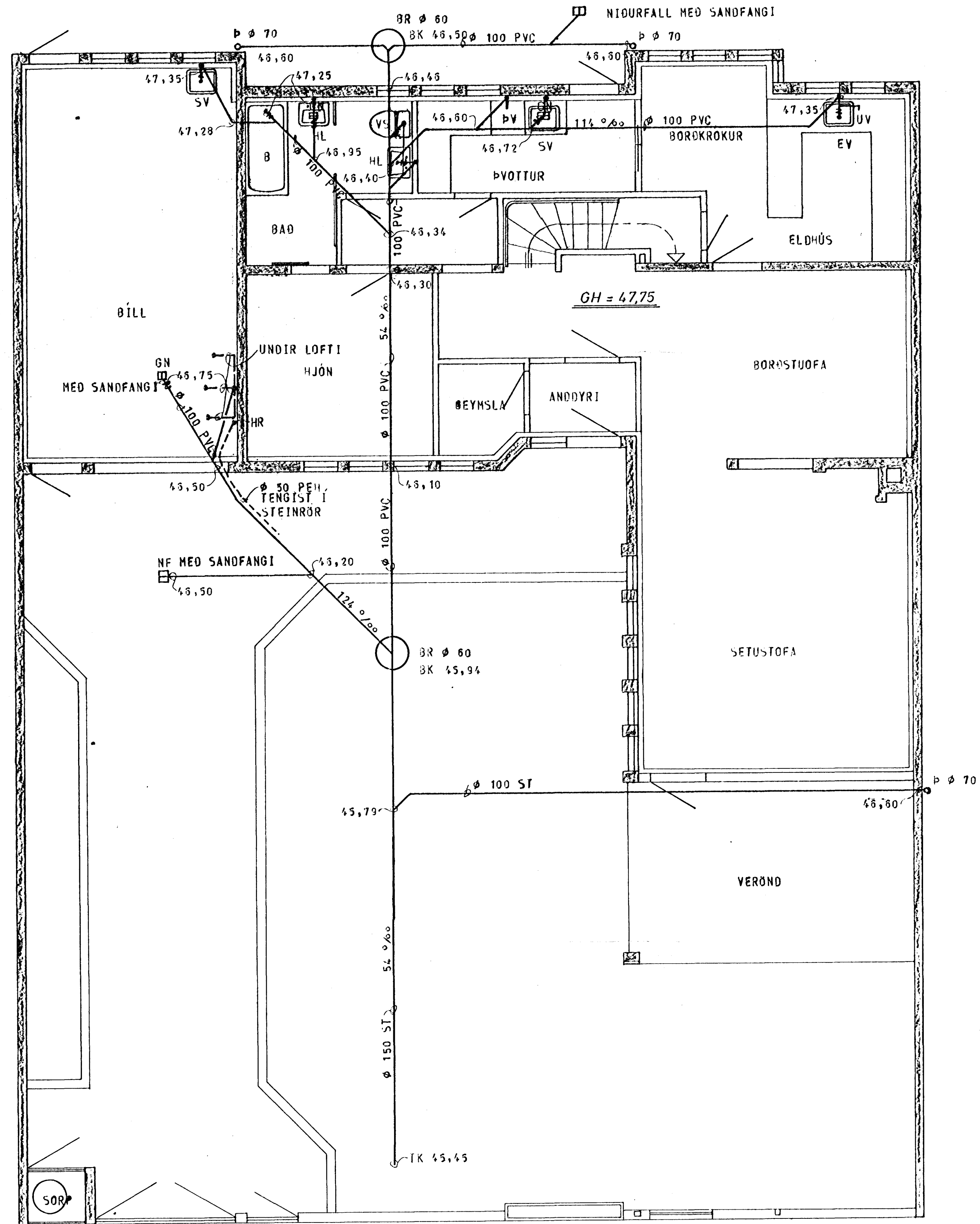
GRUNNMYND - HÆÐAR 1:50
