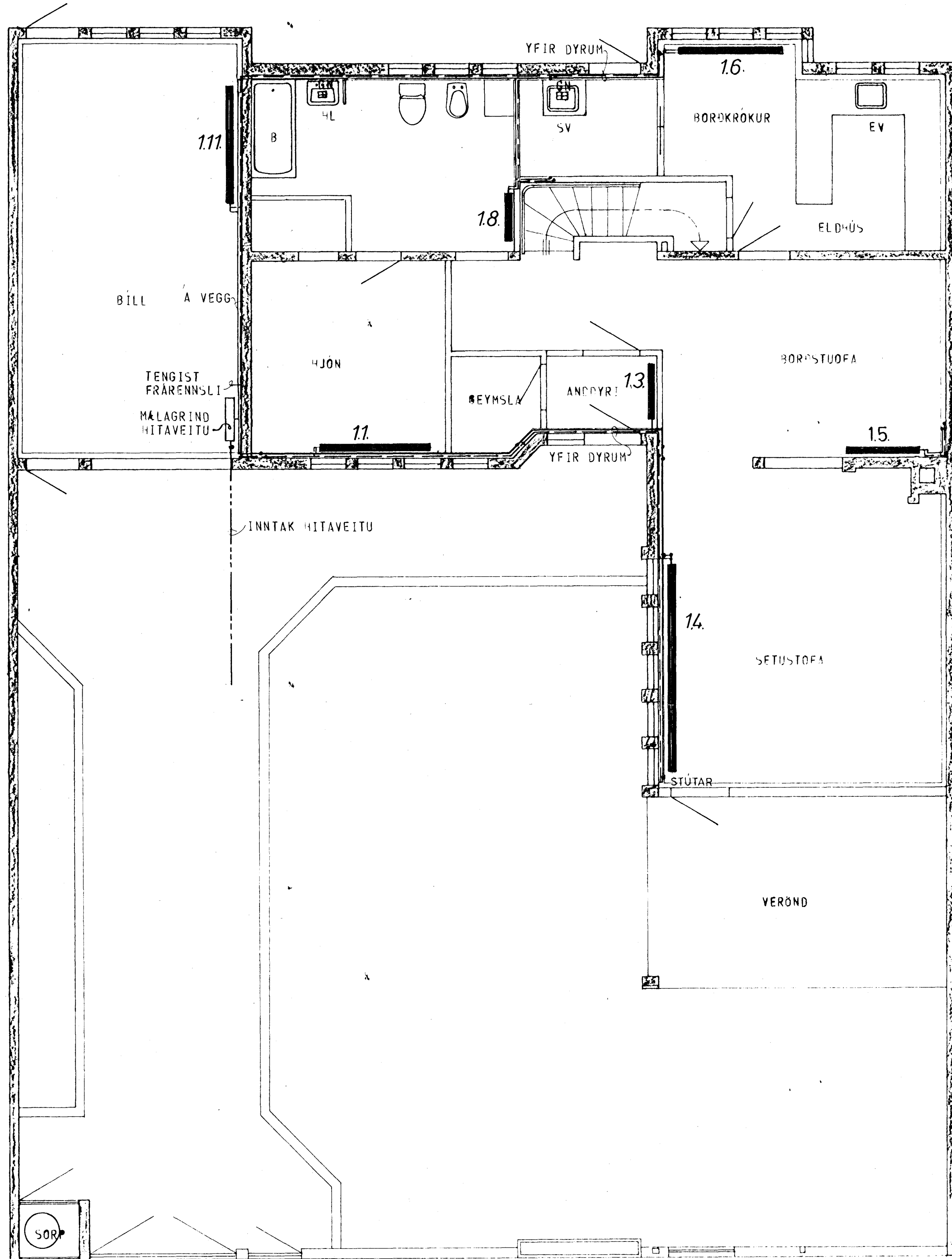
GRUNNMYND - HÆÐAR 1:50
