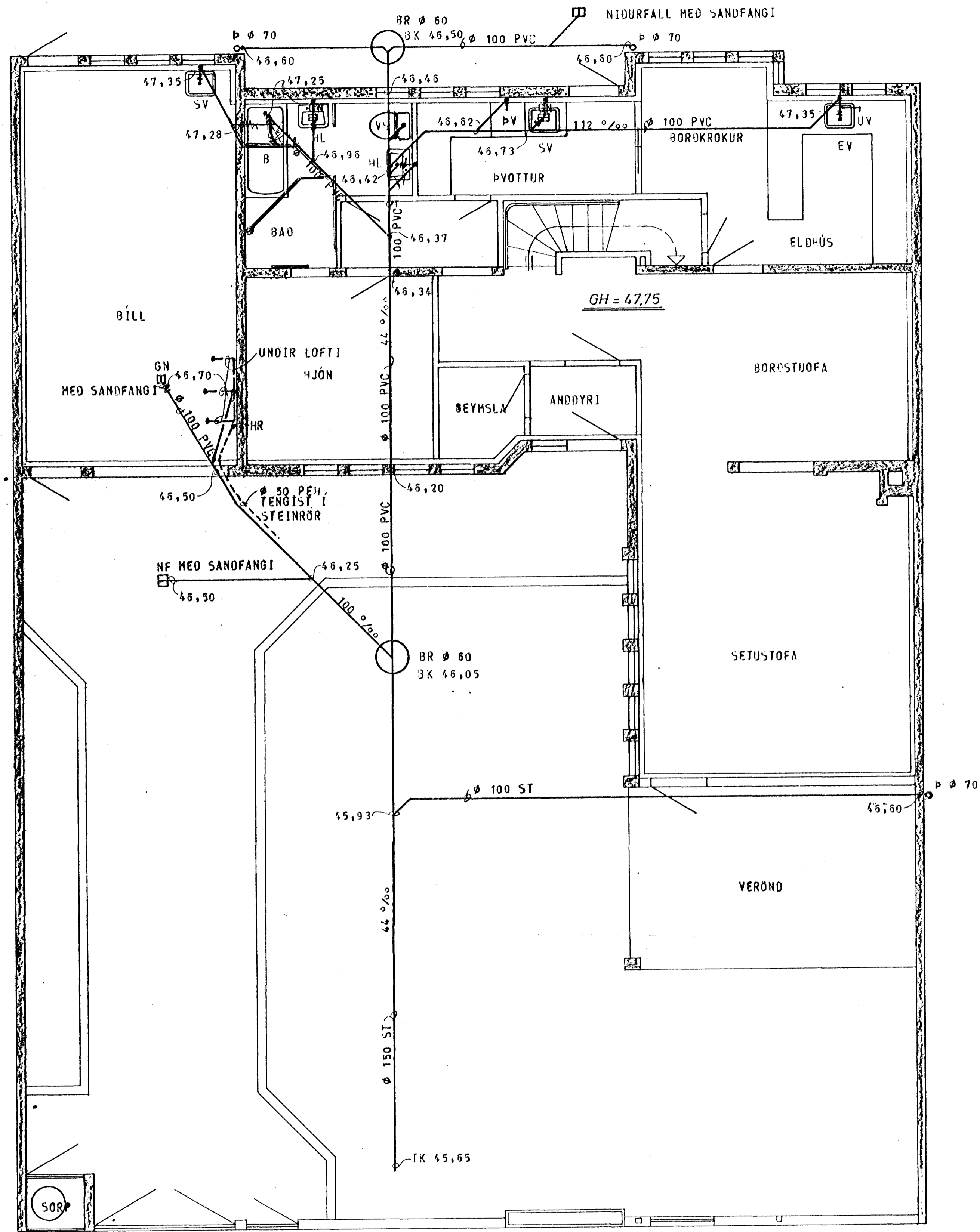
GRUNNMYND - HÆÐAR 1:50
