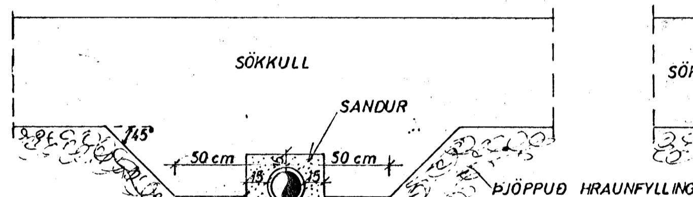
GRAFID SKAL FYRIR LÖGNUM UNDIR SÖKKLUM, AÐUR EN ÞEIR ERU STEYPTIR
